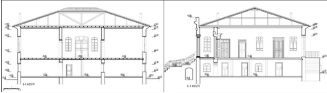
Şekil 19: 1-1 ve 2-2 kesitleri restorasyonu.
