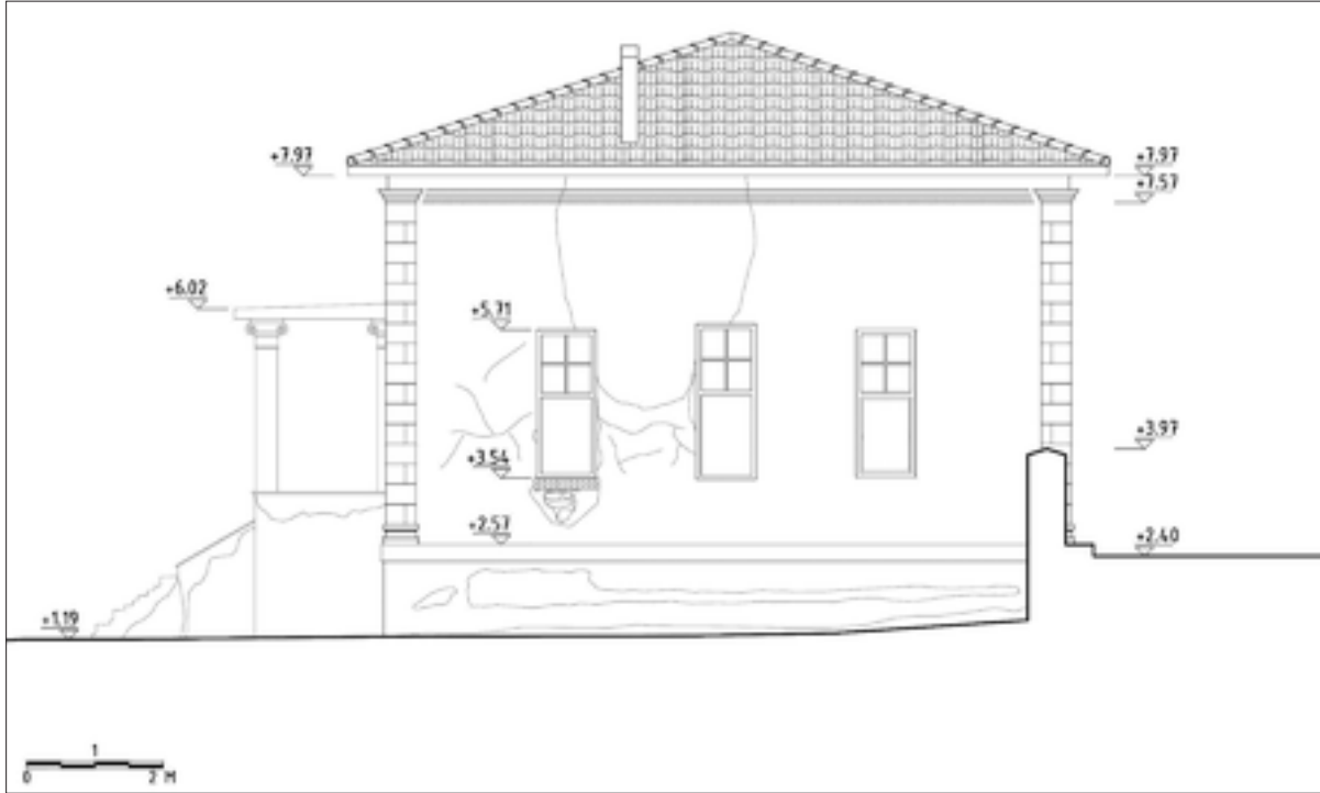
Şekil 11: Yan (batı) cephe.
