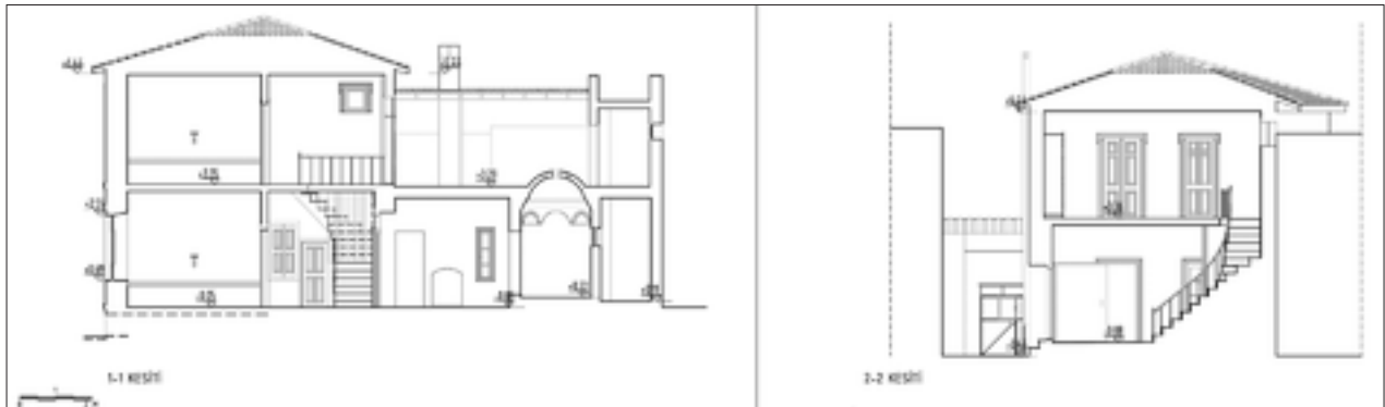
Şekil 8: Rölöve kesitler.
