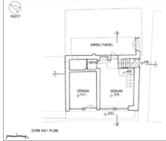
Şekil 3: Zemin kat planı.
