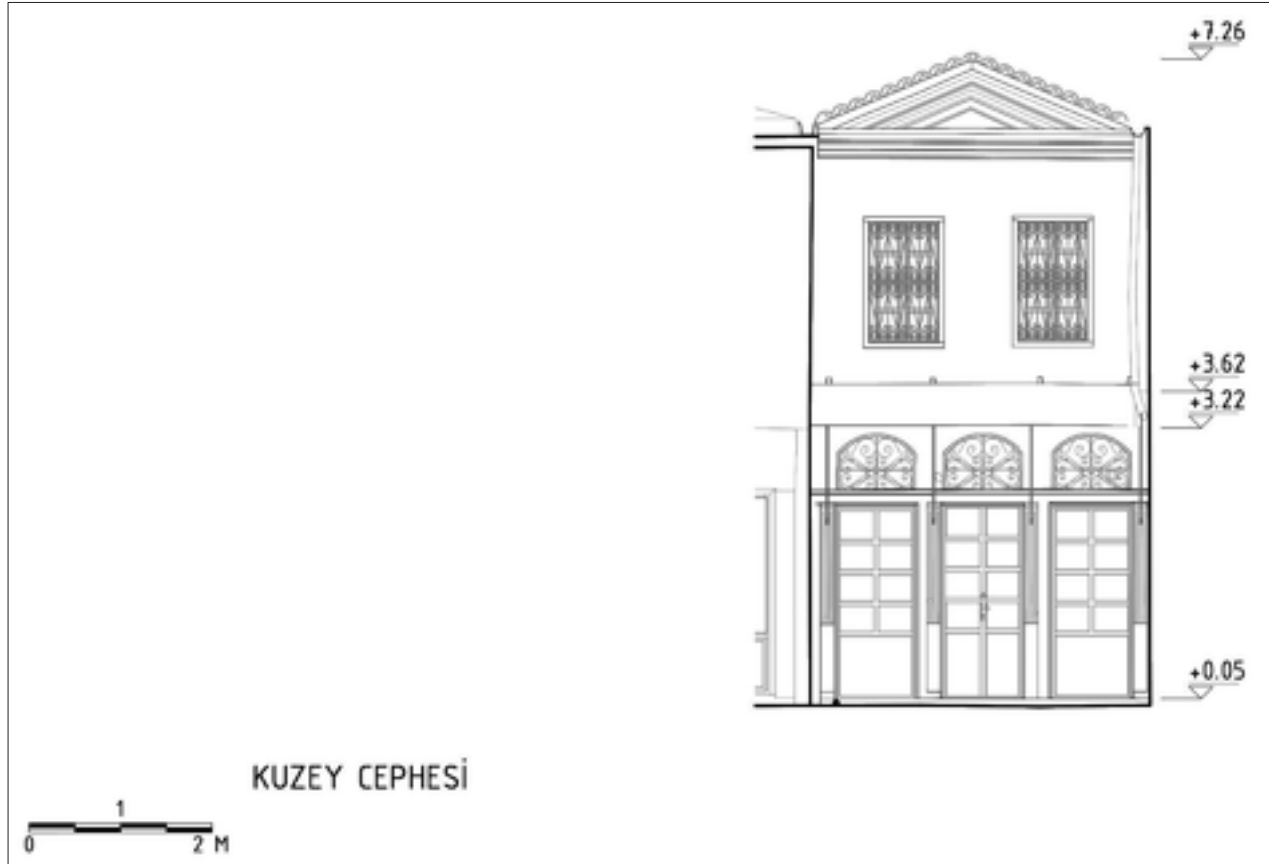
Şekil 12: Kuzey Cephesi restorasyon önerisi.
