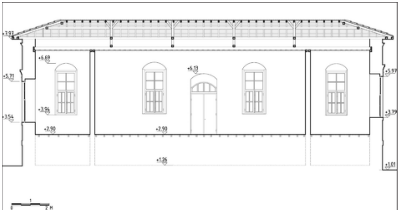
Şekil 20: Restorasyon önerisi 1-1 kesiti.
