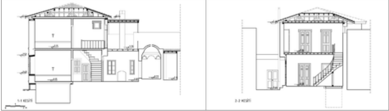
Şekil 15: Restorasyon kesitler.
