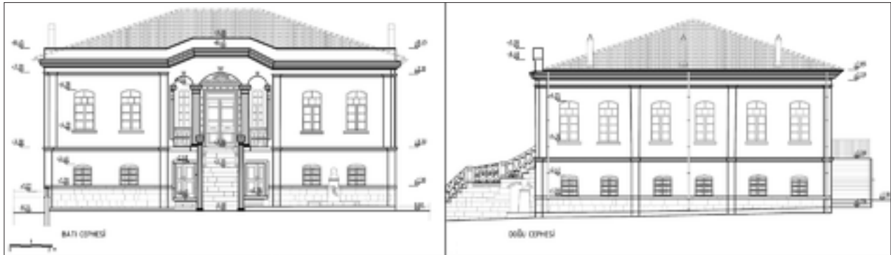
Şekil 20: Batı (giriş) ve güney (sağ yan) cepheleri restorasyonu.
