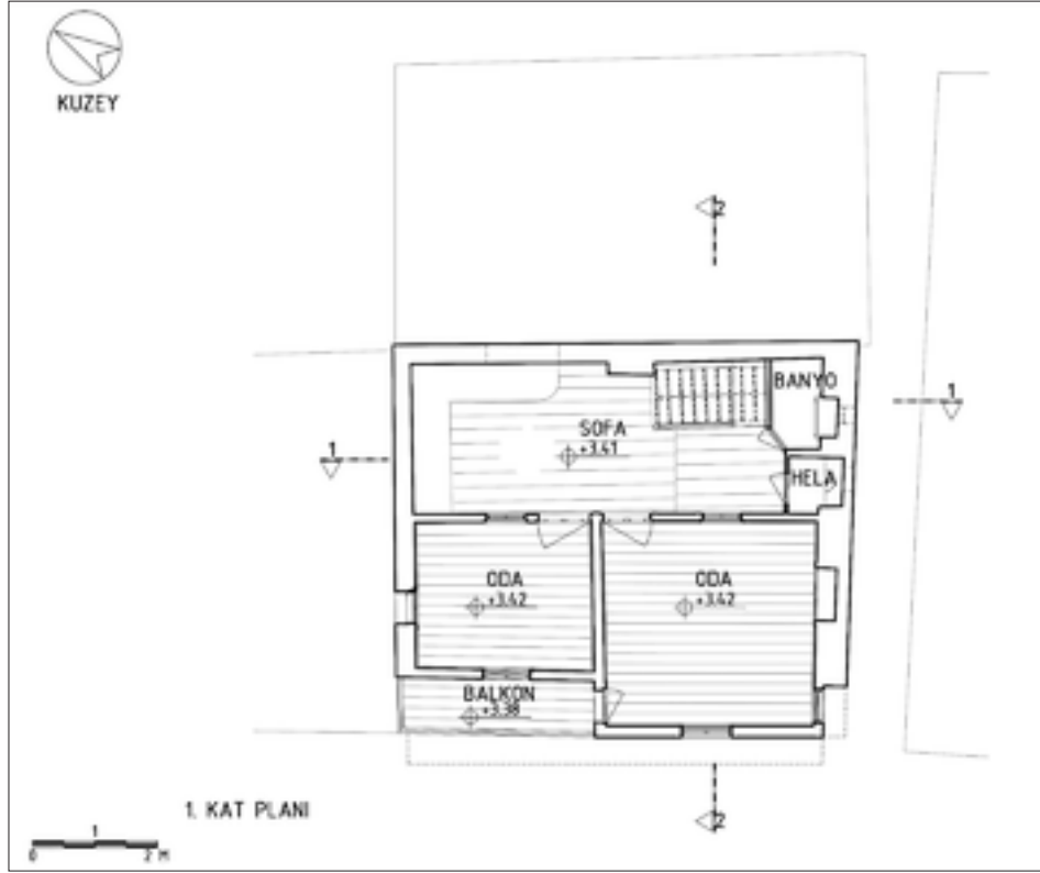
Şekil 24: Birinci kat planı restorasyon önerisi
