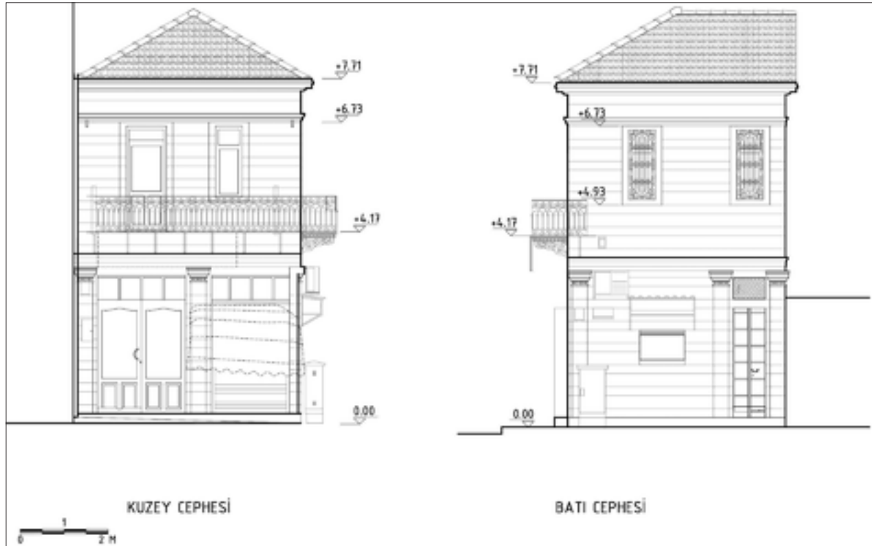
Şekil 5: Kuzey (Cumhuriyet Cad.) ve batı cephesi rölöveleri.
