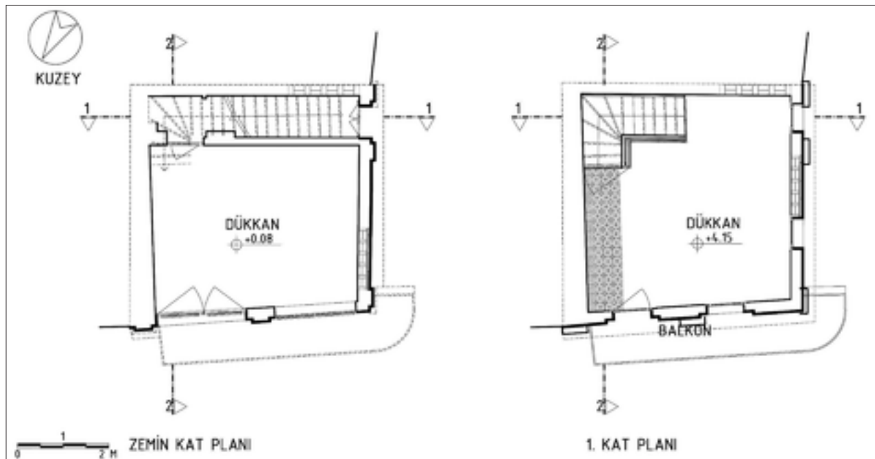
Şekil 6: Zemin ve birinci kat restitüsyon planları.
