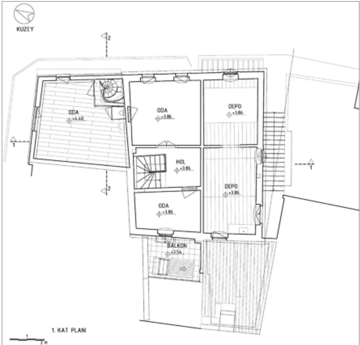
Şekil 10: Birinci kat rölöve planı.
