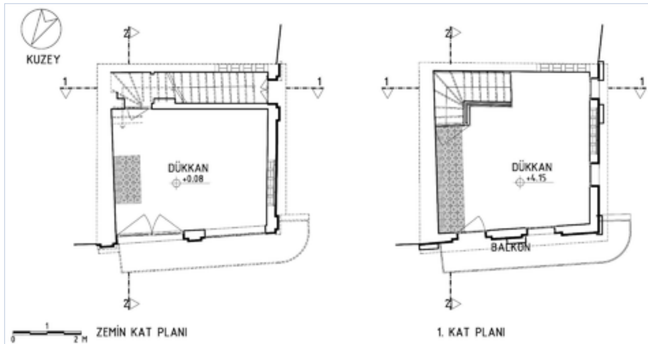
Şekil 9: Zemin ve birinci kat restorasyon planları.
