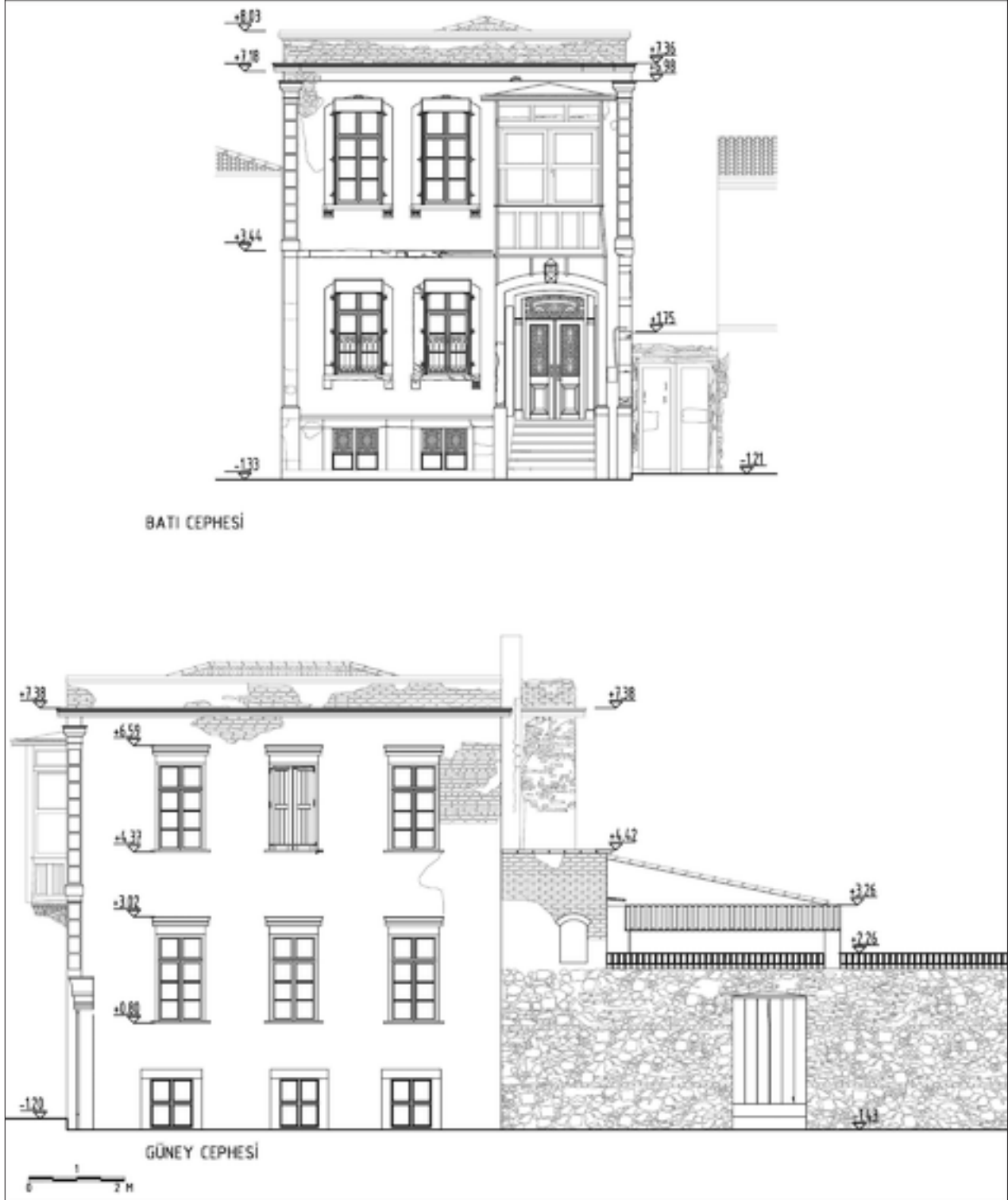
Şekil 9: Rölöve cepheler.
