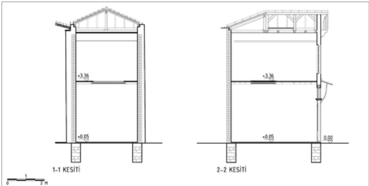
Şekil 8: Restitüsyon enine ve boyuna kesit.
