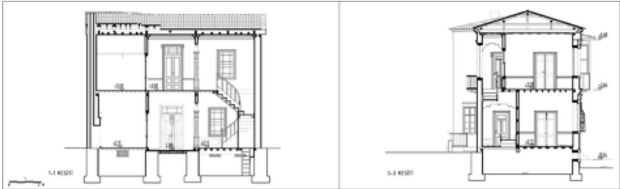
Şekil 15: 1-1 ve 3-3 kesitleri I. dönem restitüsyon önerileri.
