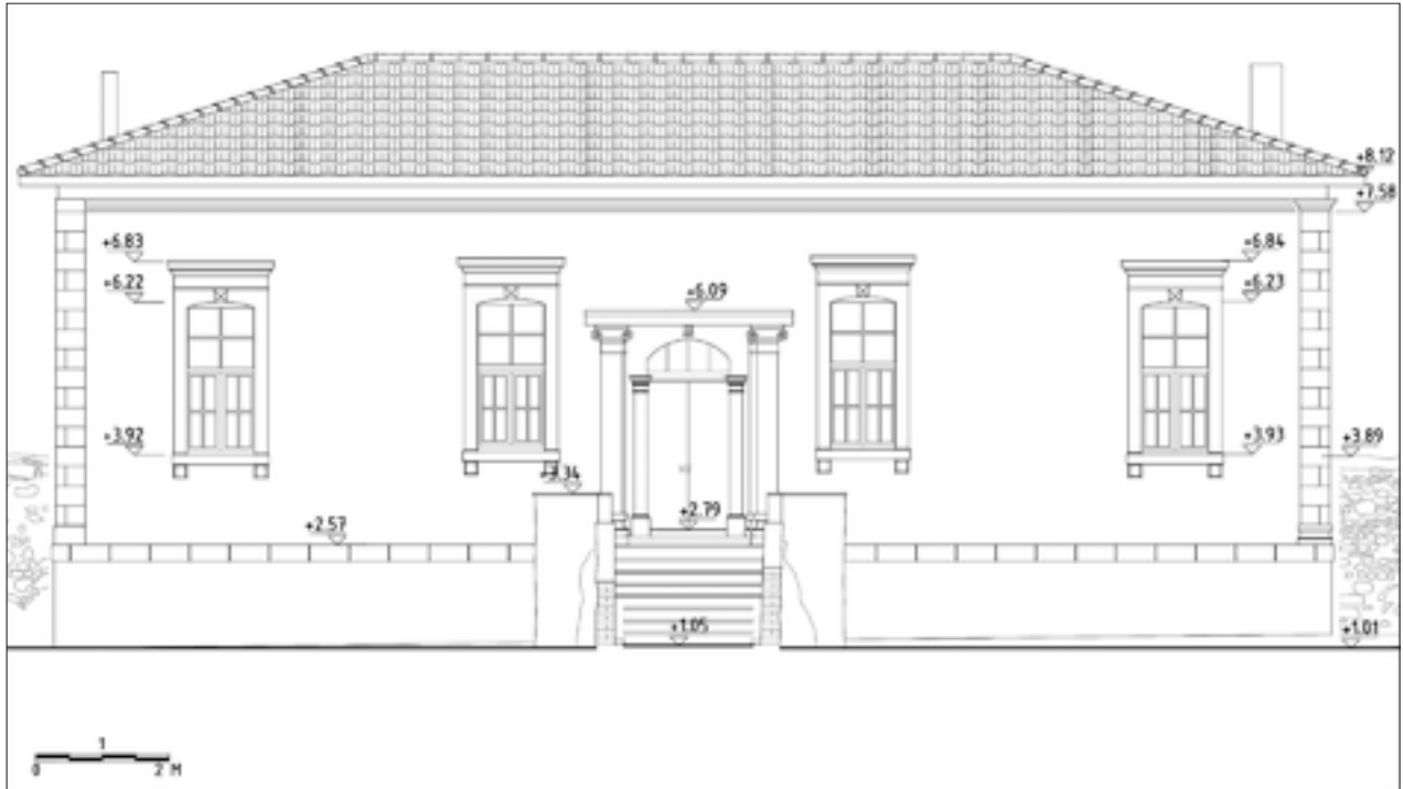
Şekil 22: Restorasyon önerisi ön (kuzey) cephe.
