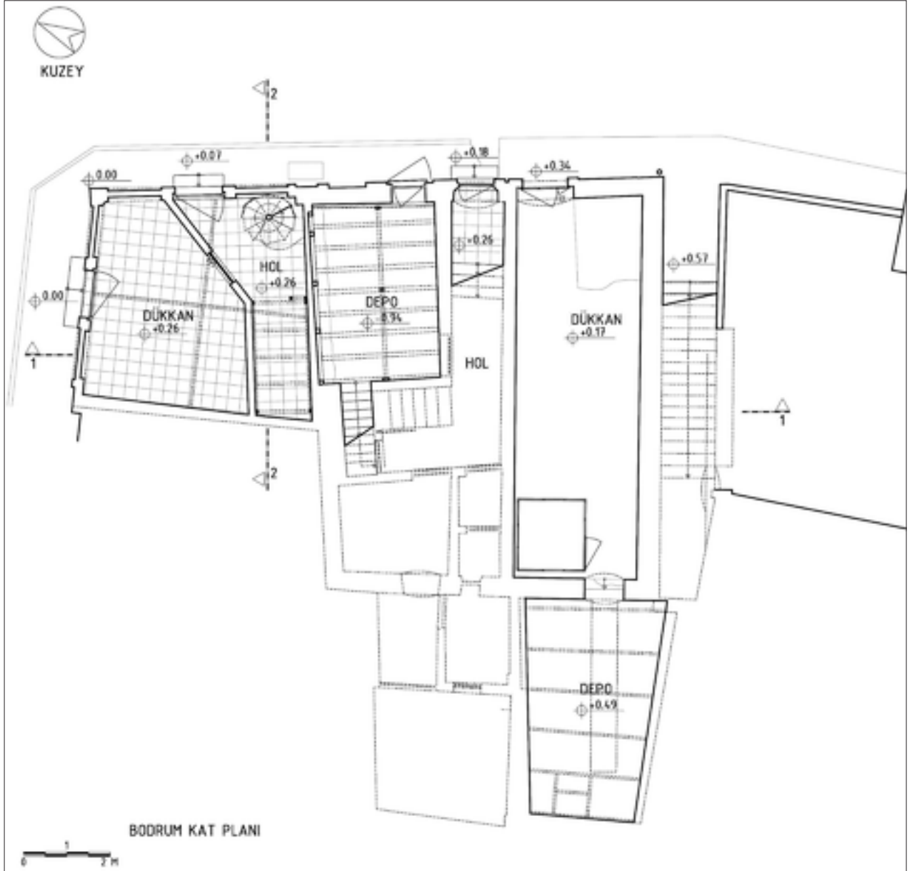
Şekil 8: Bodrum kat rolöve planı.
