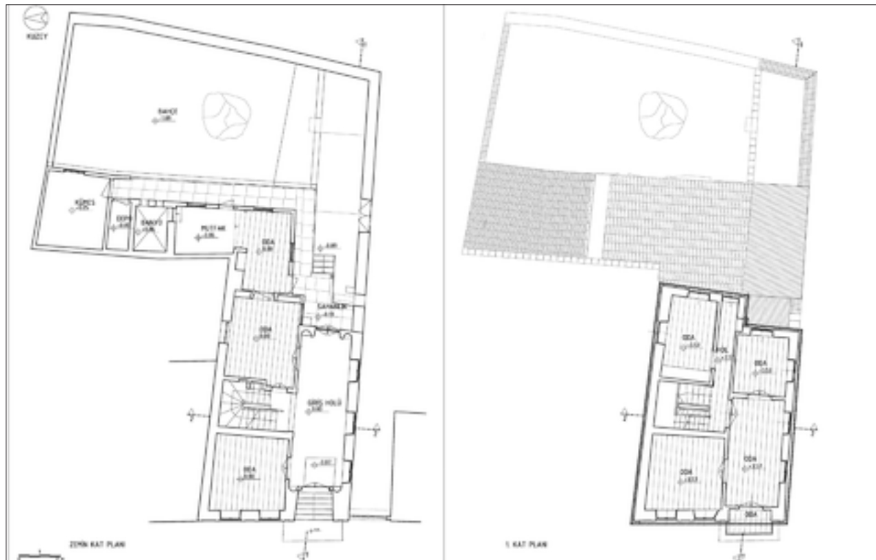
Şekil 7: Rölöve zemin ve 1. kat planı.
