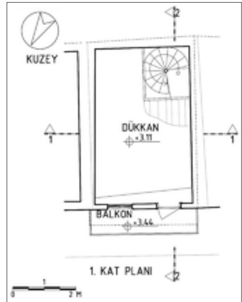
Şekil 5: 1. Kat planı.
