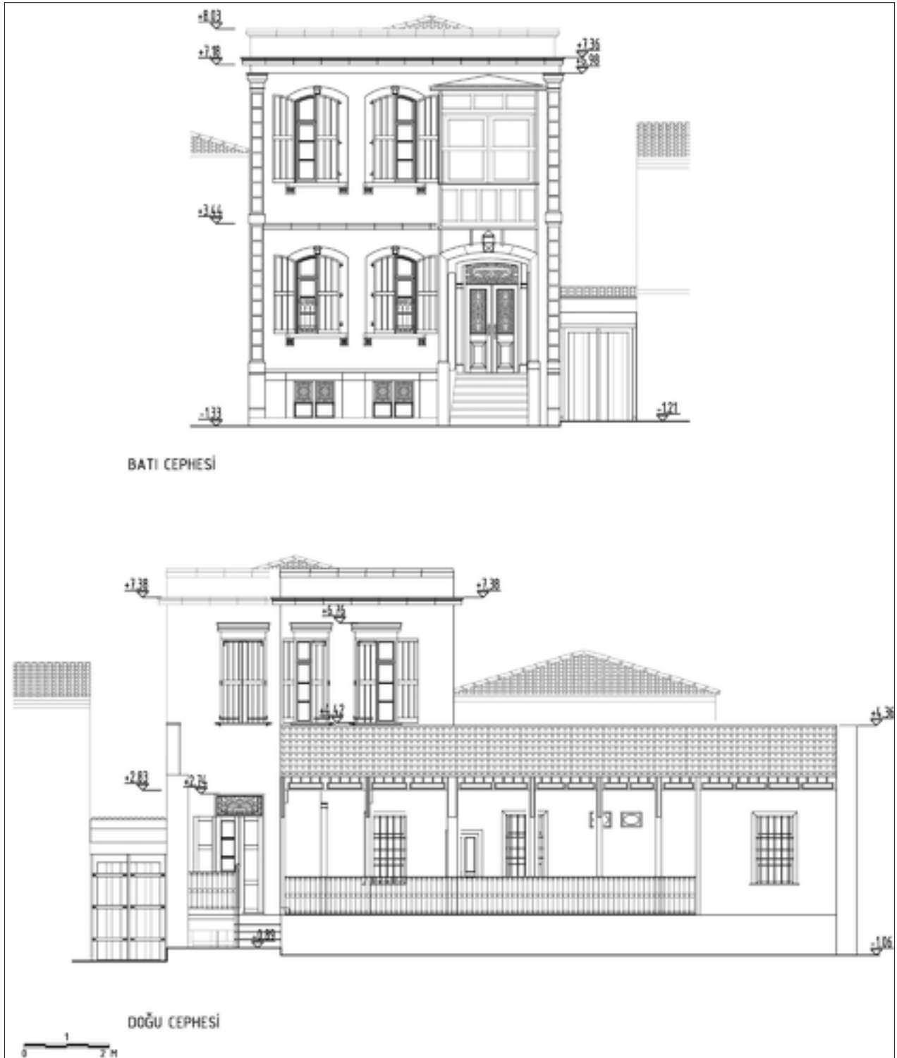
Şekil 11: Restitüsyon cepheler.
