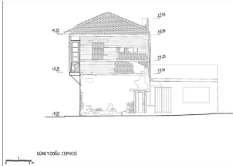
Şekil 14: Güney cephe rölöve çizimi.
