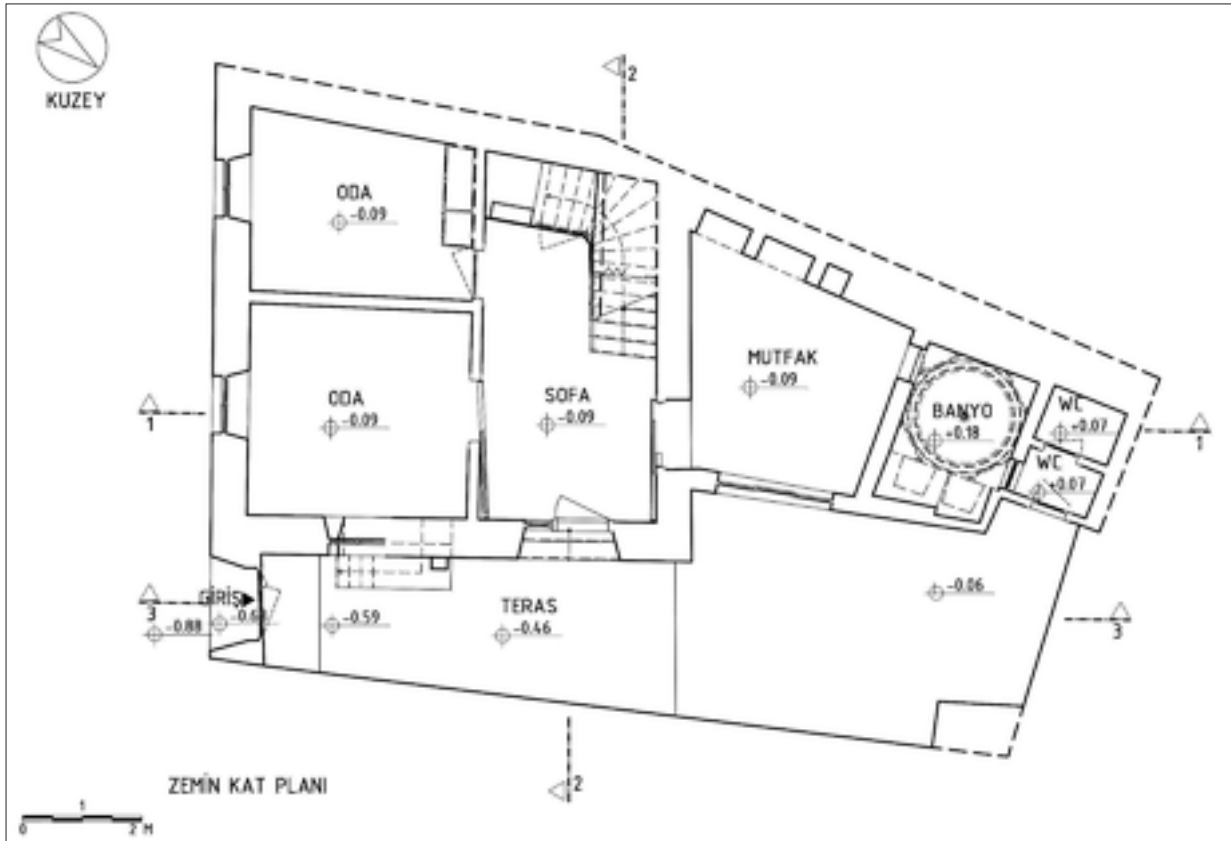
Şekil 5: Rölöve zemin kat planı.
