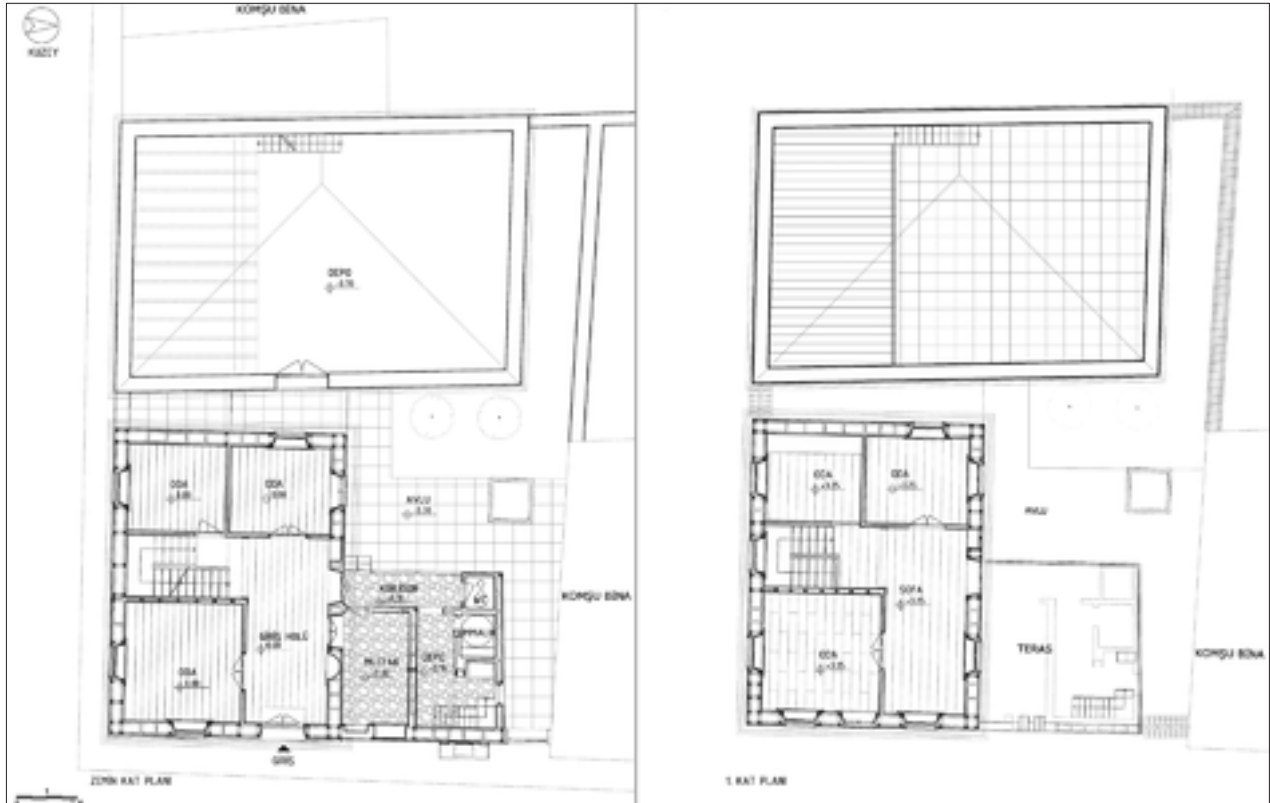
Şekil 10: Restitüsyon zemin ve 1. kat planları.
