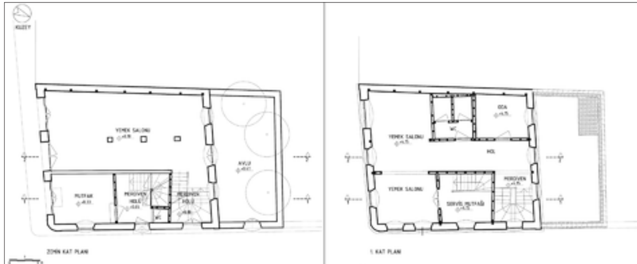
Şekil 12: Restorasyon kat planları.
