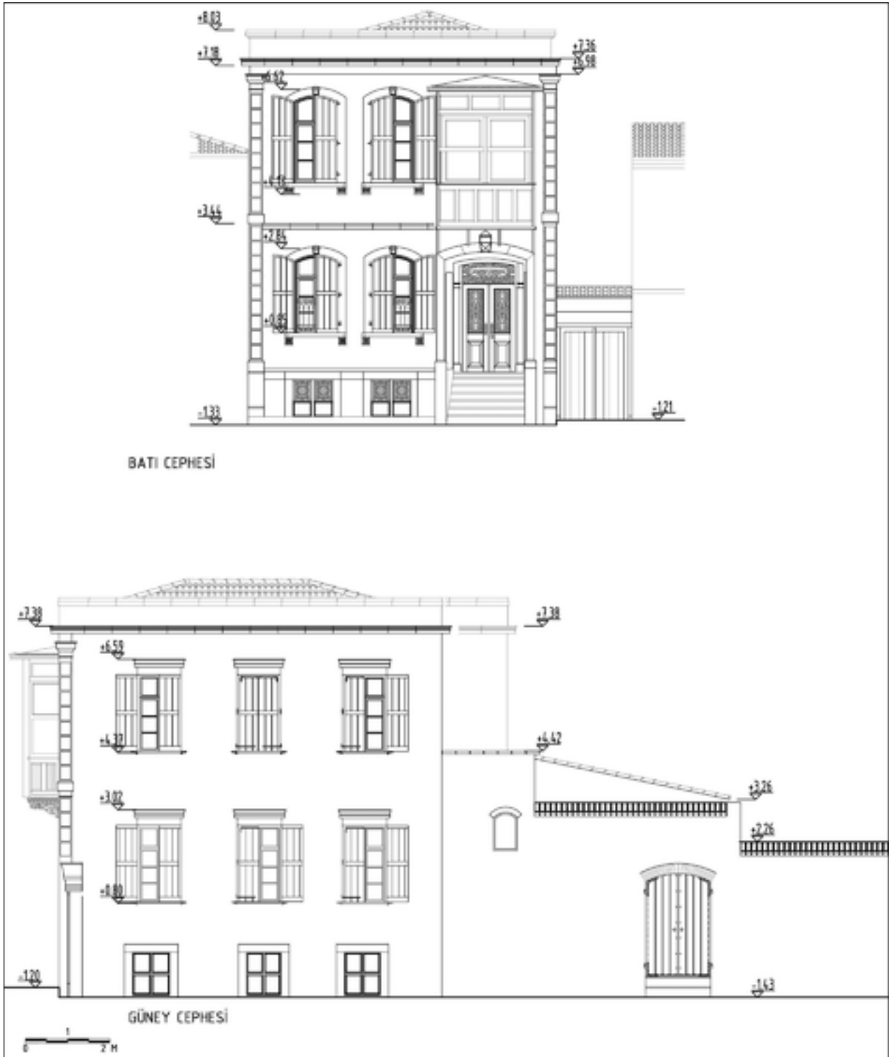
Şekil 14: Restorasyon cepheler.
