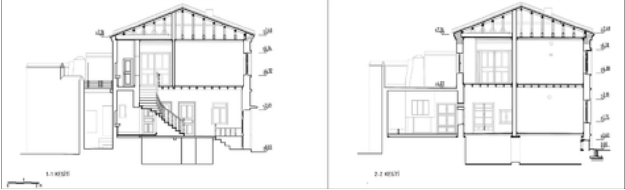
Şekil 10: Restorasyon enine ve boyuna kesit.
