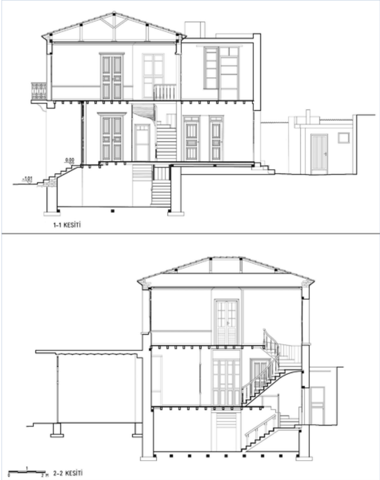
Şekil 17: 2. dönem restitüsyon - boyuna kesitler.
