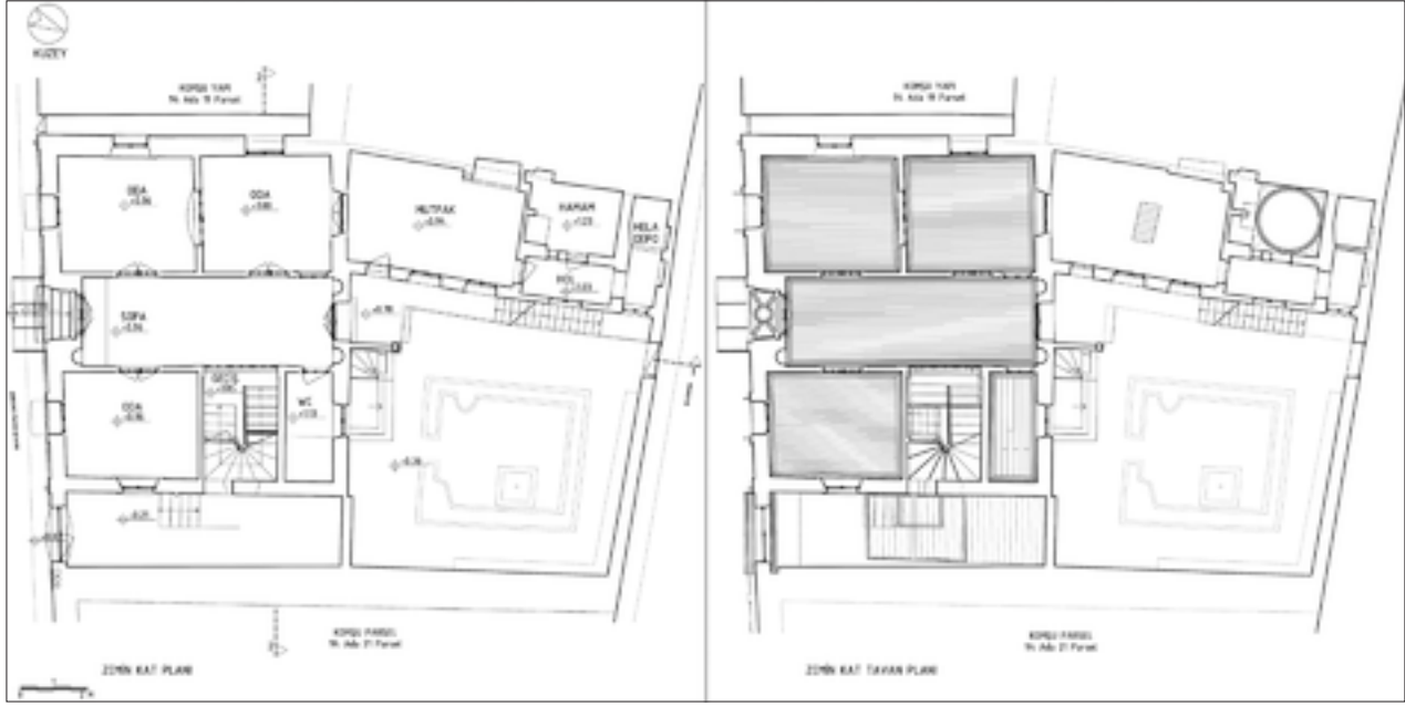
Şekil 5: Rölöve zemin kat ve tavan planı.
