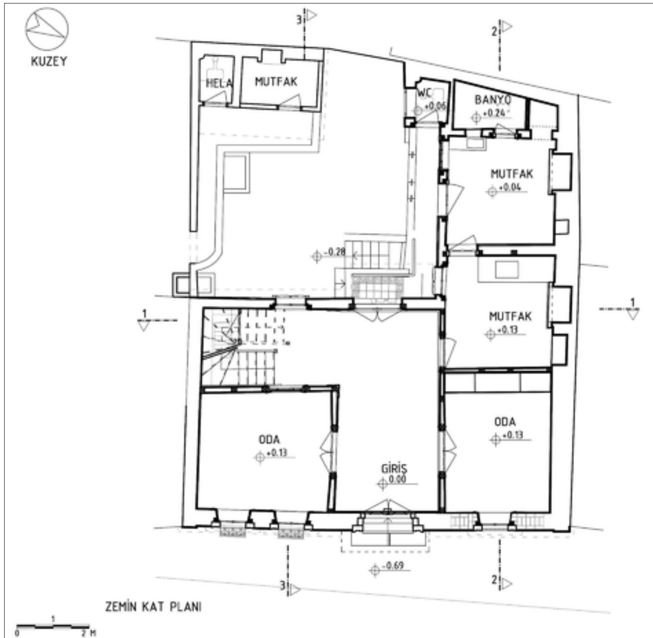
Şekil 17: Zemin kat planı II. dönem restitüsyon önerisi.
