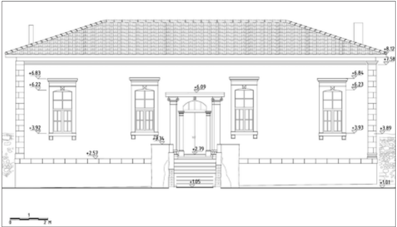
Şekil 16: Restitüsyon projesi ön (kuzey) cephe.
