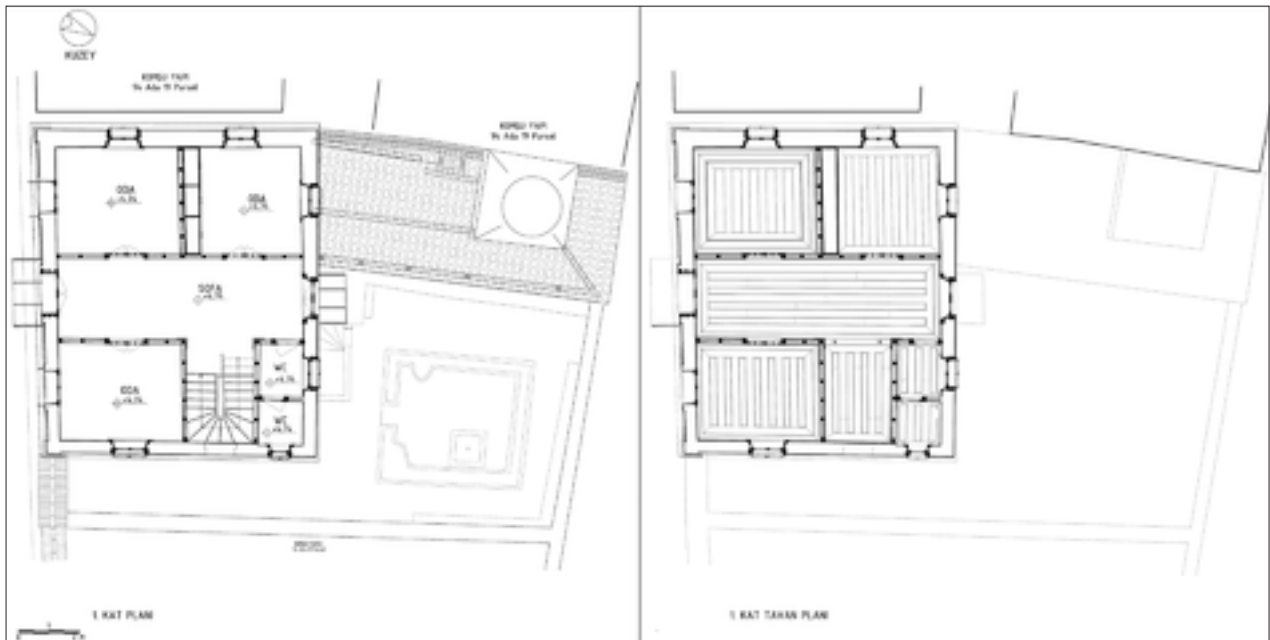
řekil 21: Restorasyon 1. kat ve tavan planı.
