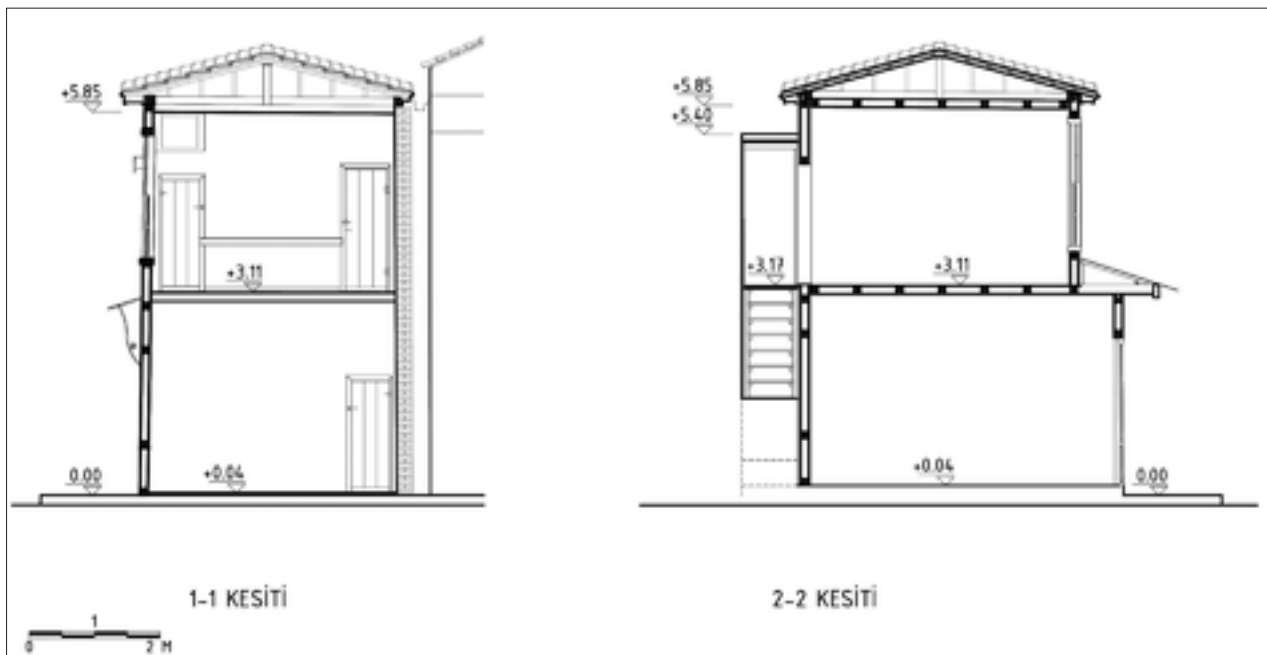
Şekil 13: Restorasyon enine ve boyuna kesit.
