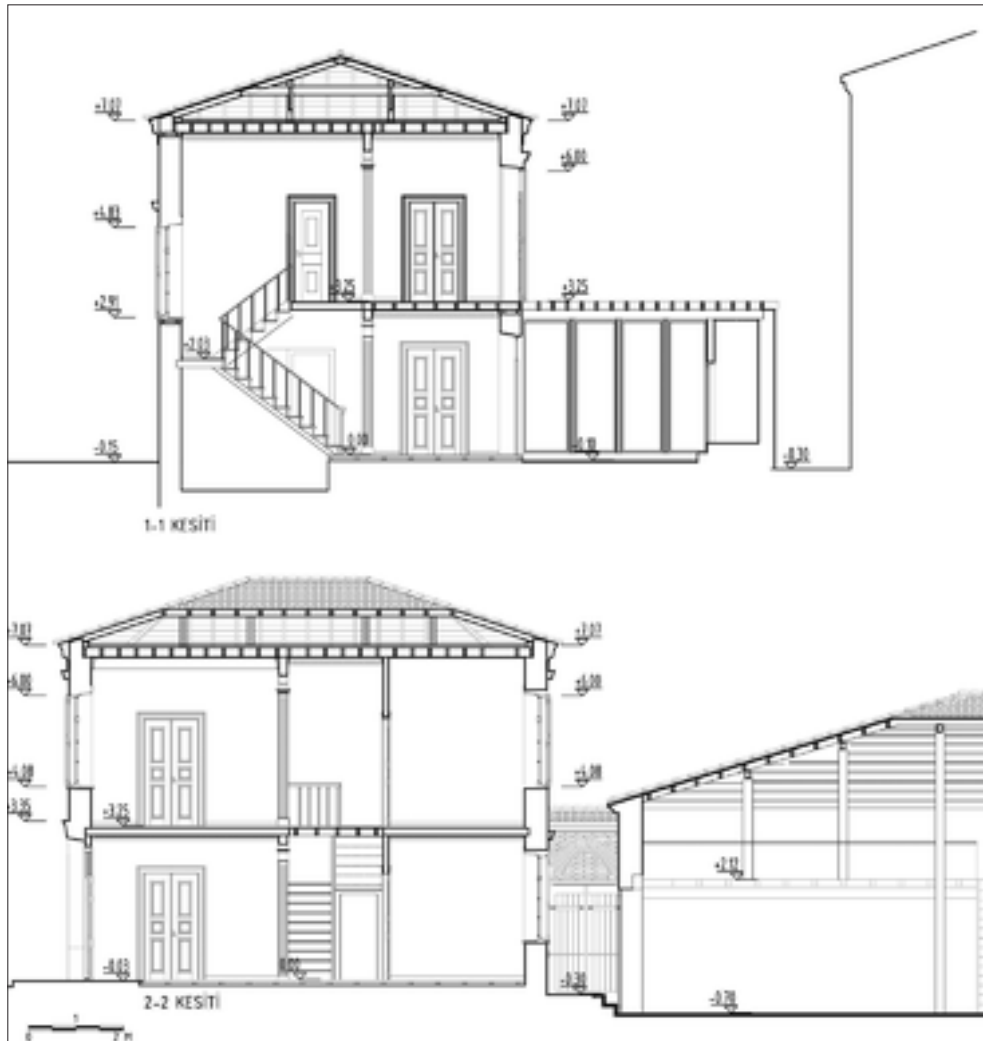
Şekil 14: Restorasyon kesitler.
