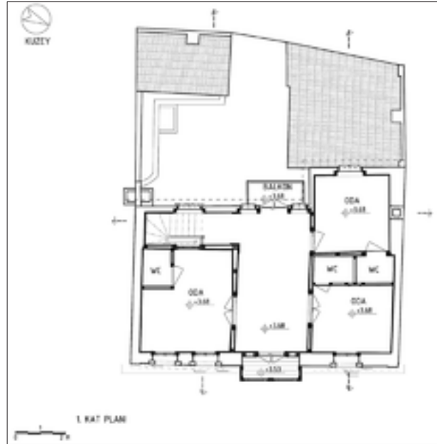
Şekil 22: Birinci kat restorasyon önerisi.
