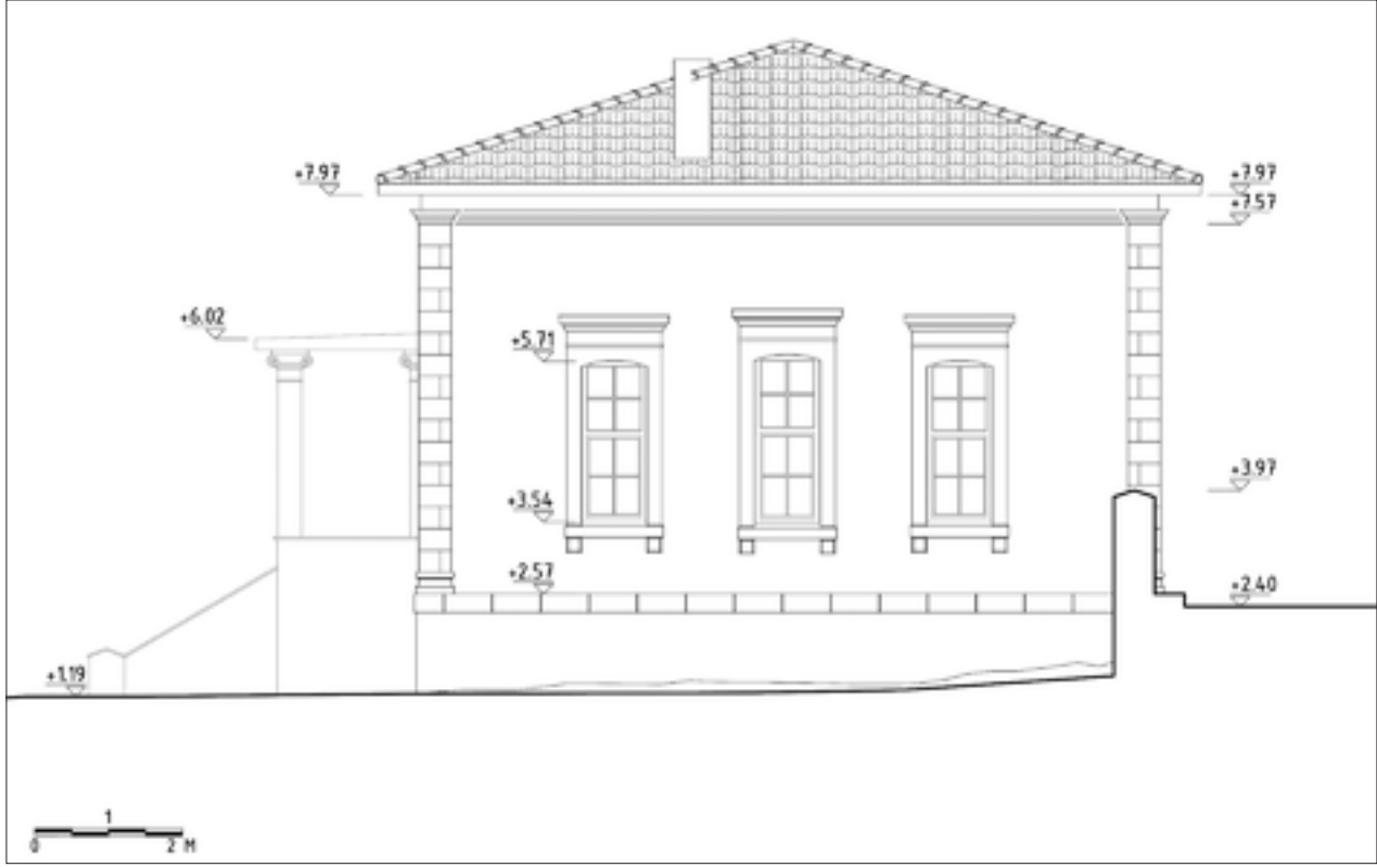
Şekil 17: Restitüsyon projesi yan (batı) cephe.
