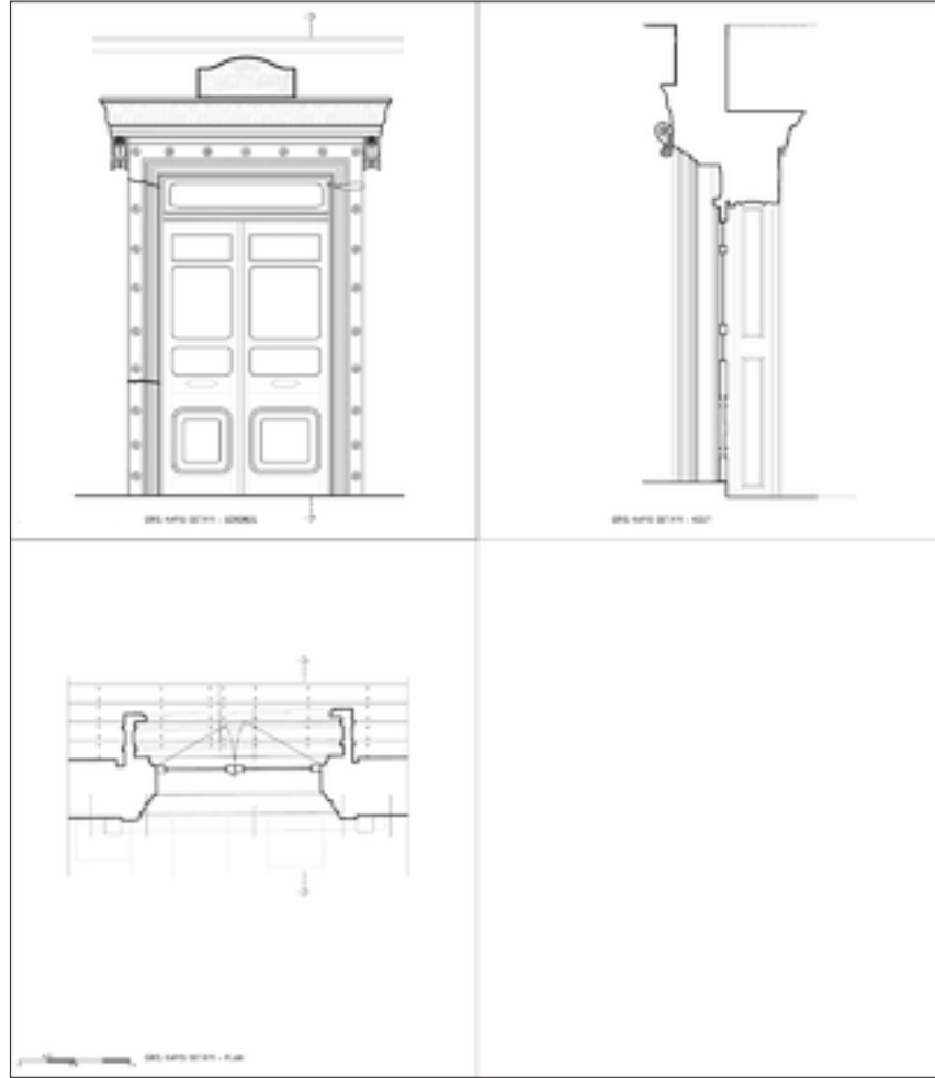
Şekil 8: Birinci kat giriş kapısı detayı rölövesi.
