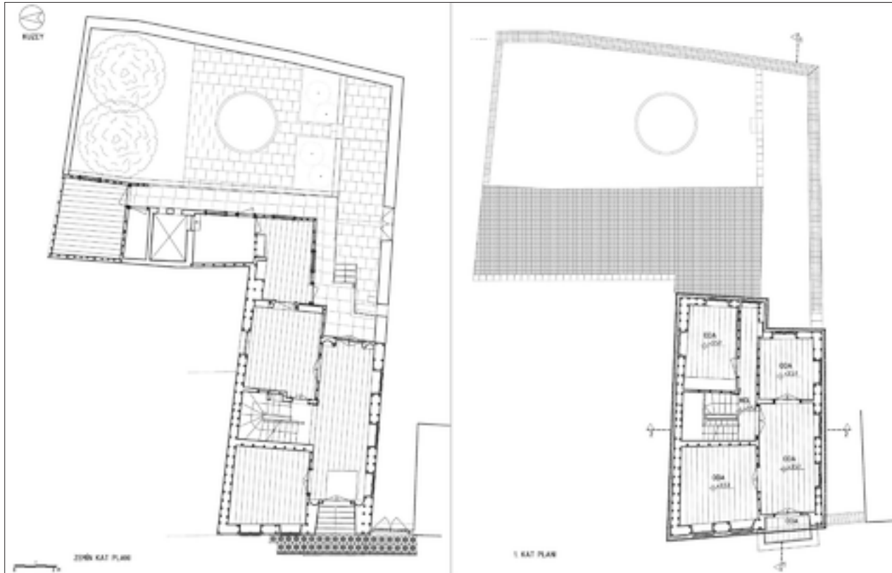
Şekil 10: Restitüsyon planları.
