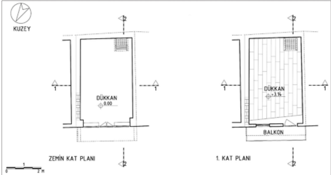
Şekil 8: Restitüsyon kat plan önerileri.
