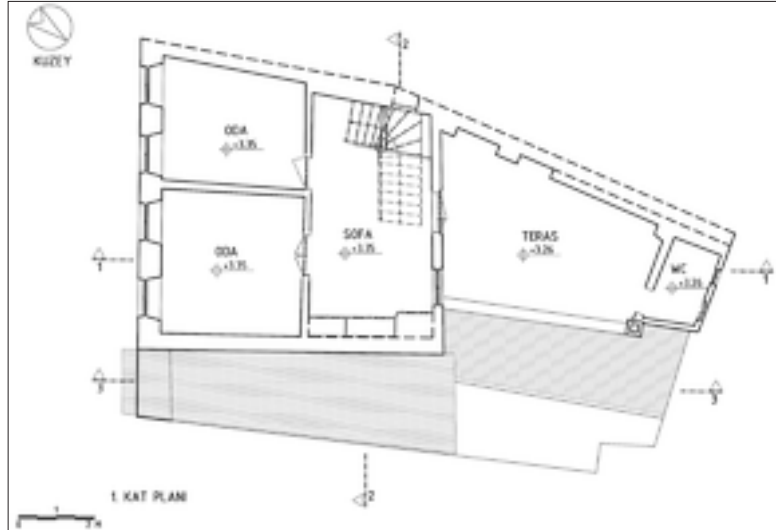
Şekil 7: Rölöve 1. kat planı.
