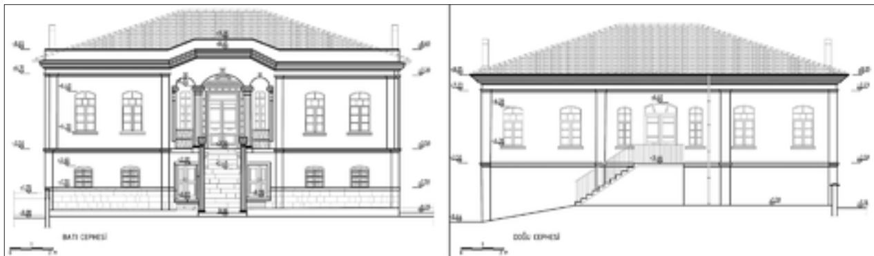
Şekil 15: Batı (giriş) ve doğu cepheleri restitüsyon önerisi.
