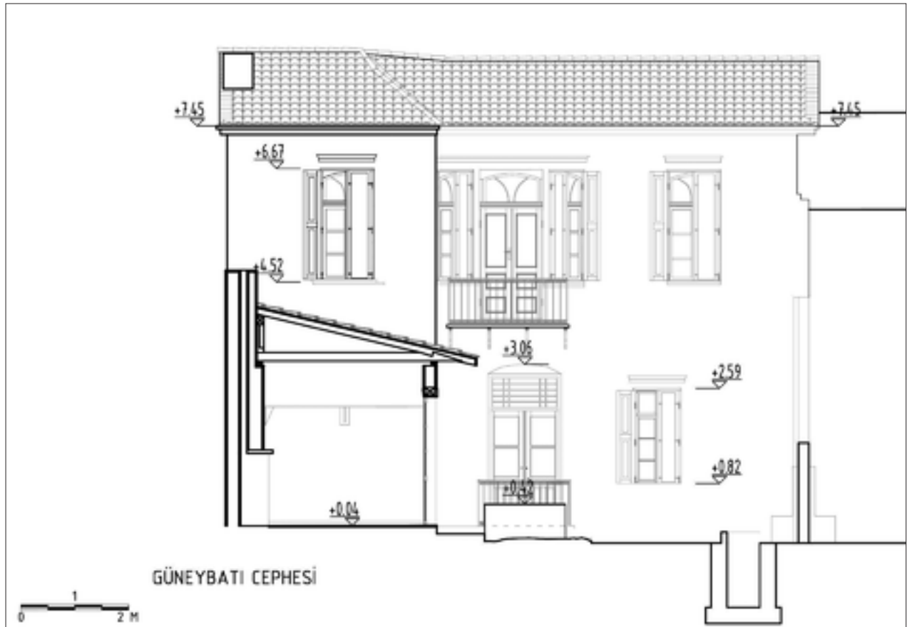
Şekil 20: Arka Cephe restorasyon önerisi.
