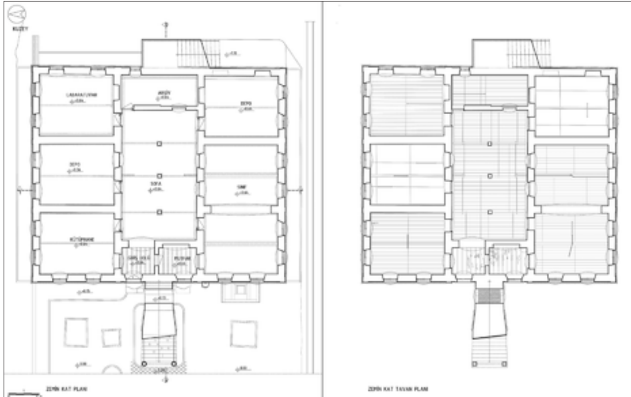
Şekil 4: Zemin kat plan ve tavan rölövesi.
