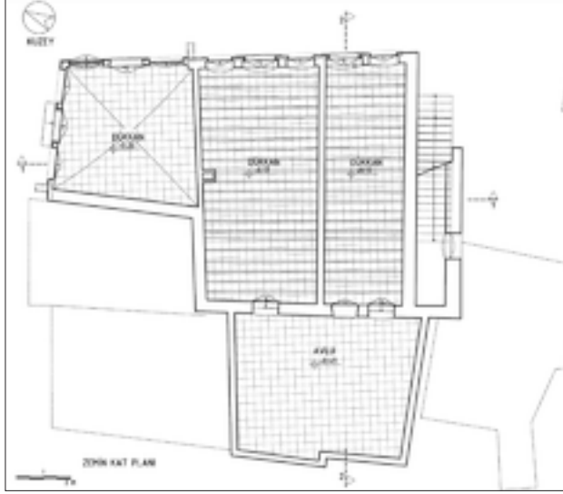
Şekil 14: Zemin kat restitüsyon planı.
