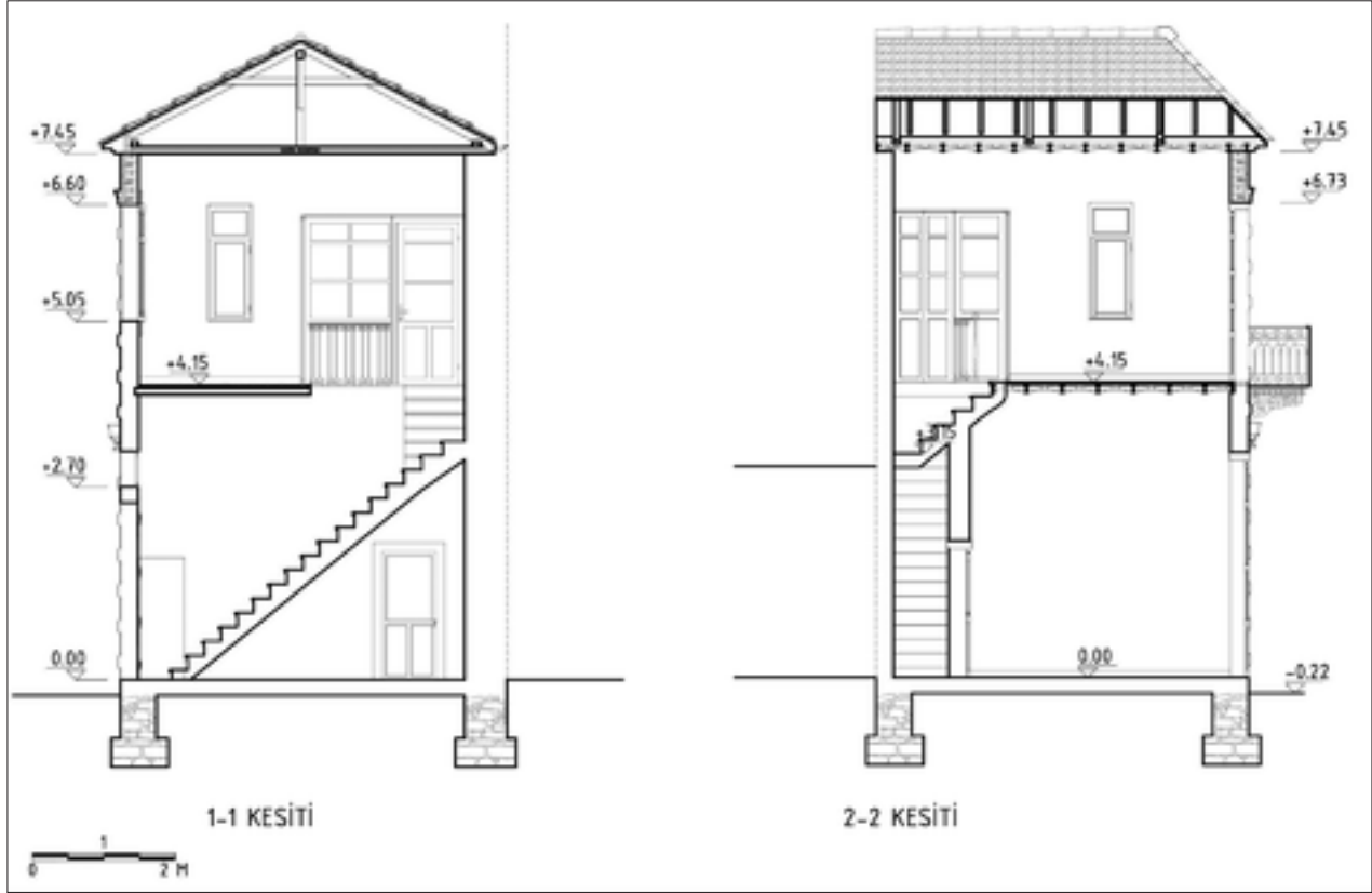
Şekil 10: Restorasyon kesitler.
