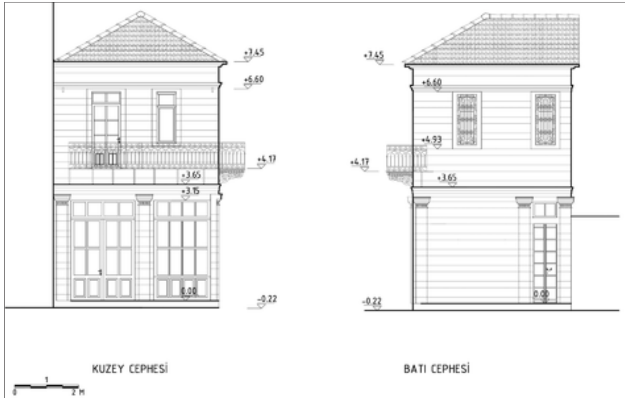
Şekil 8: Kuzey (Cumhuriyet Caddesi) ve batı cephesi restitüsyon cepheleri.
