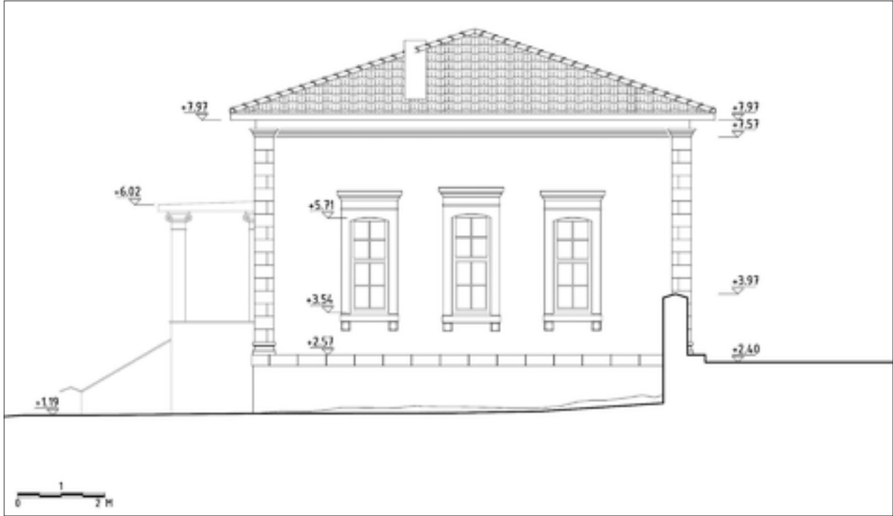
Şekil 23: Restorasyon önerisi yan (batı) cephe.
