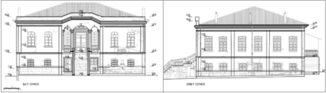
Şekil 7: Batı (giriş) ve güney (sağ yan) rölöve cepheleri.
