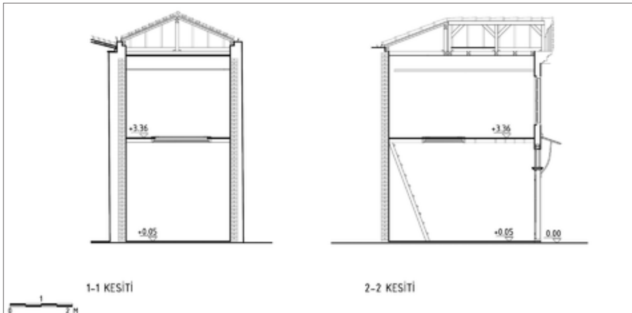
Şekil 11: Restorasyon kesitler.
