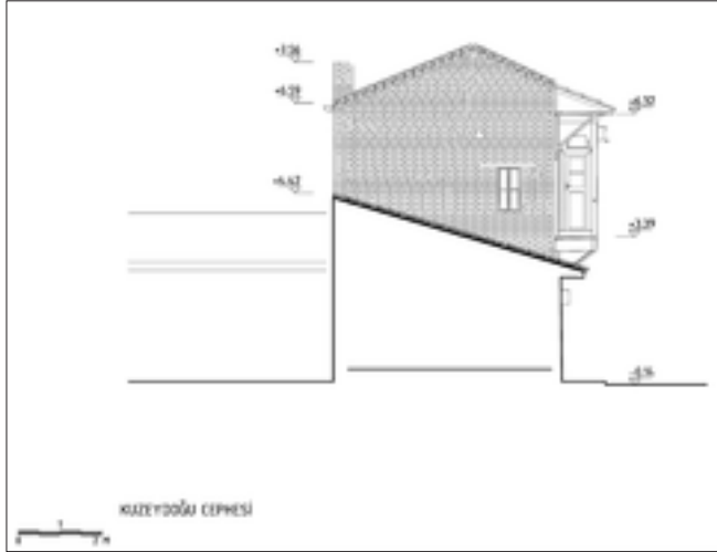
Şekil 16: Kuzey cephesi rölöve çizimi.
