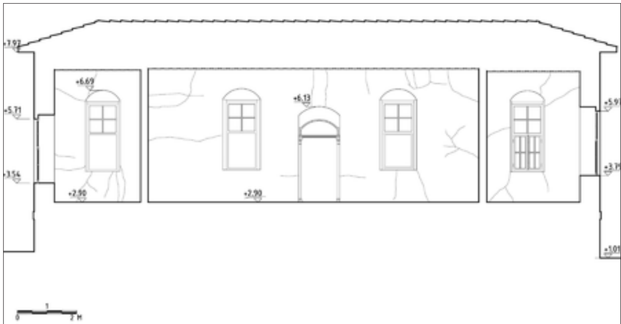
Şekil 8: 1-1 Kesiti.
