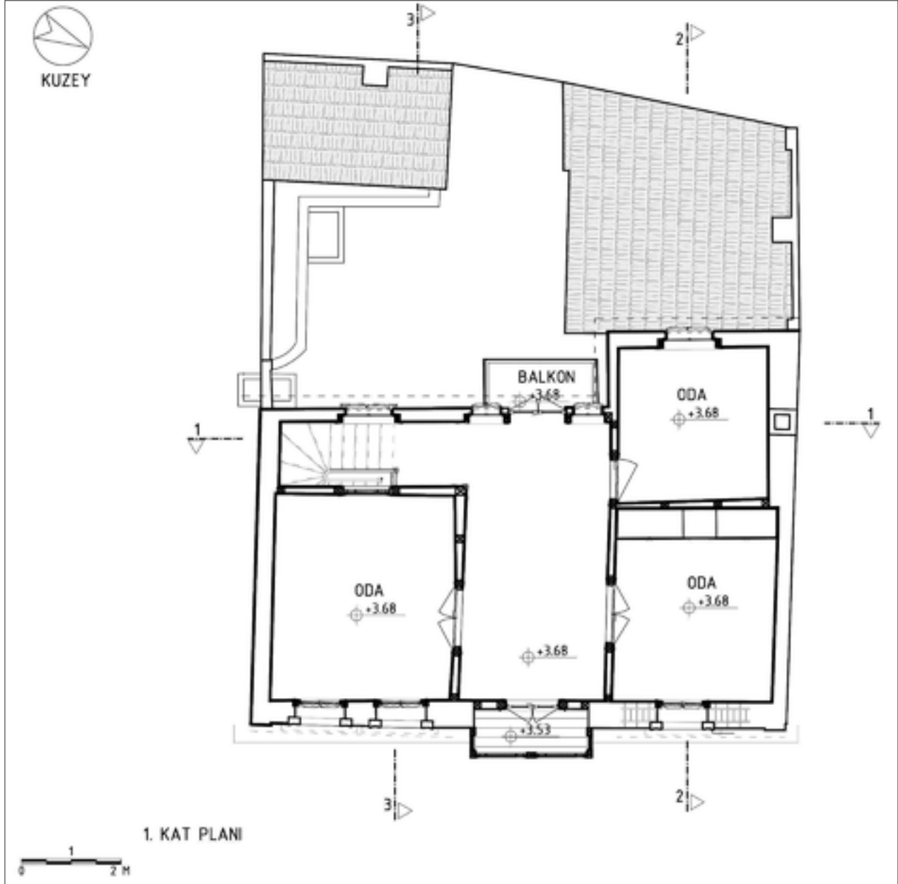
Şekil 18: Birinci kat planı II. dönem restitüsyon önerisi.
