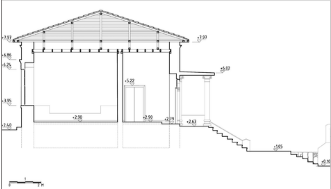
Şekil 21: Restorasyon önerisi 2-2 kesiti.
