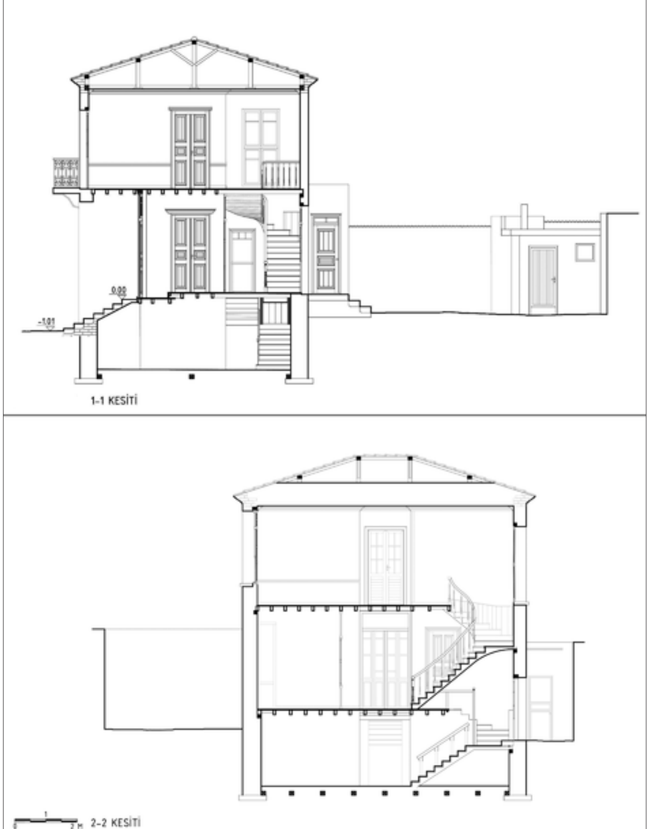
Şekil 14: 1. Dönem restitüsyon kesitler.
