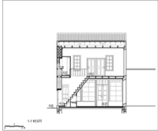
Şekil 21: 1-1 Kesiti
