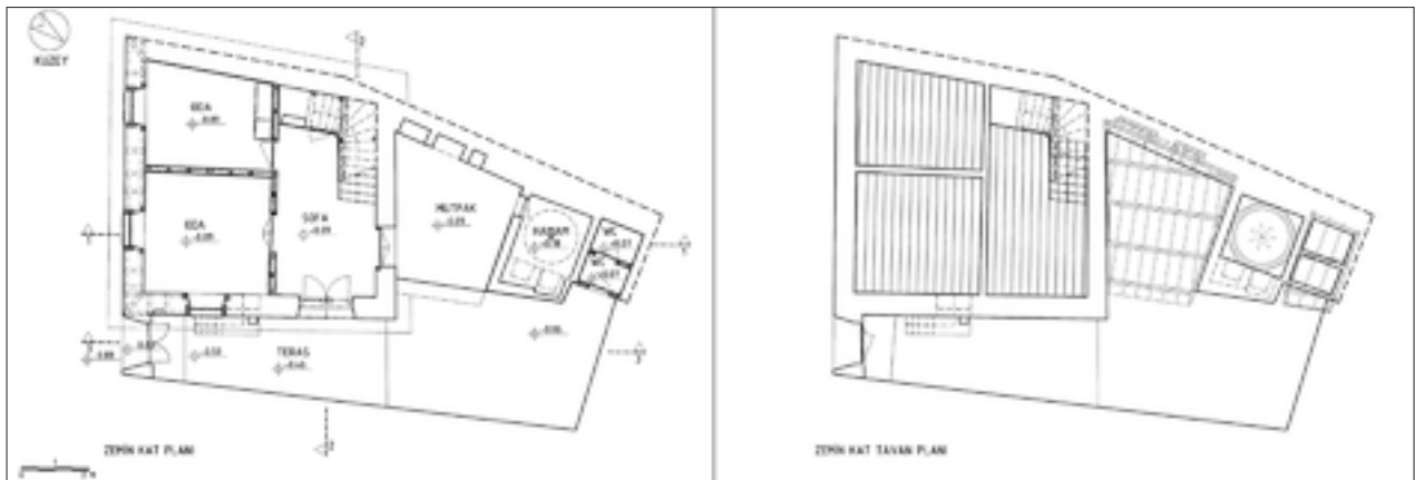
Şekil 10: Restitüsyon zemin kat ve tavan planları.
