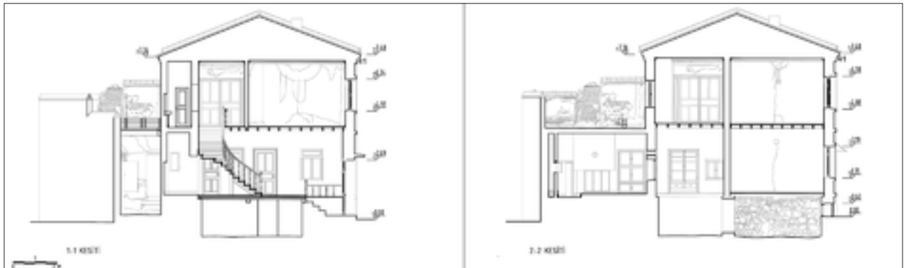
Şekil 4: Rölöve enine ve boyuna kesit.
