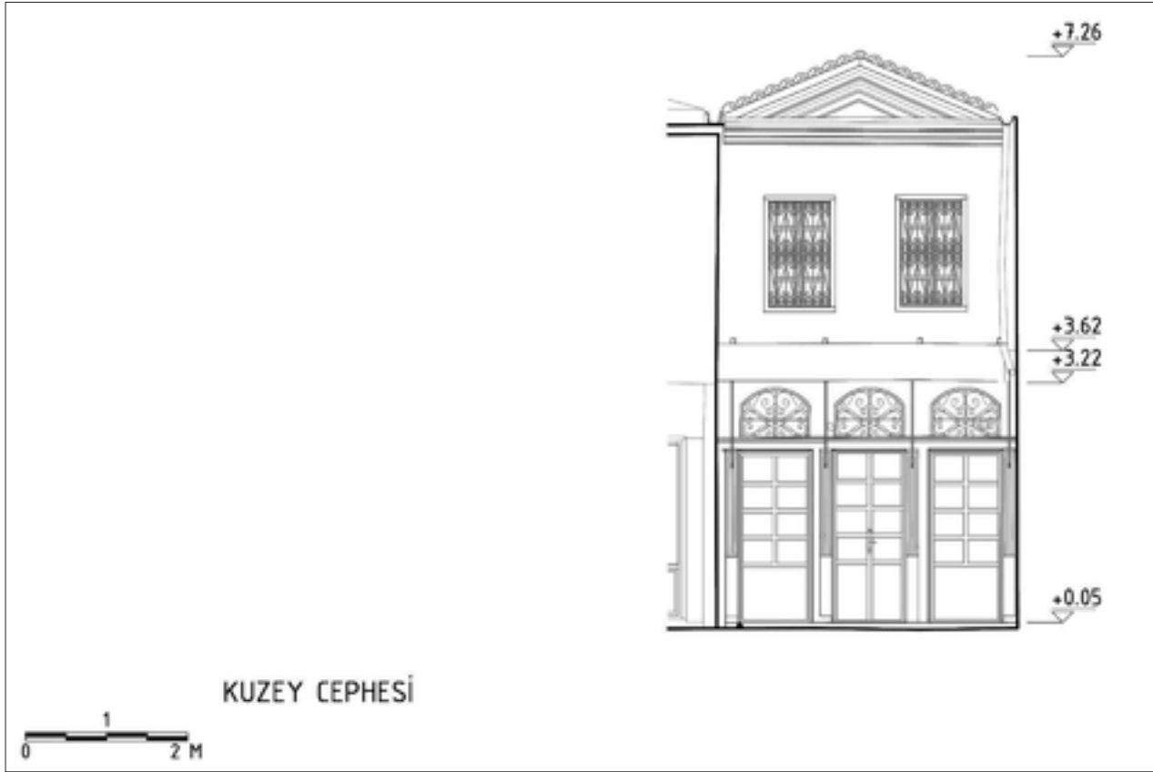
Şekil 9: Kuzey cephesi restitüsyon önerisi.
