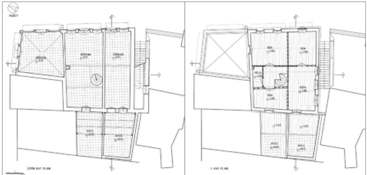
Şekil 19: Restorasyon zemin kat ve 1. kat planı.
