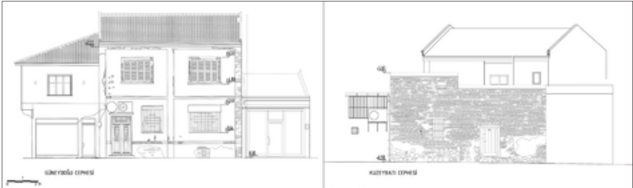
Şekil 5: Rölöve cepheler.
