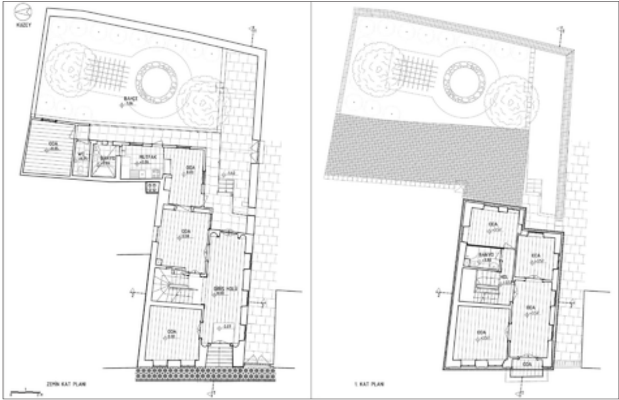
Şekil 12: Restorasyon kat planları.
