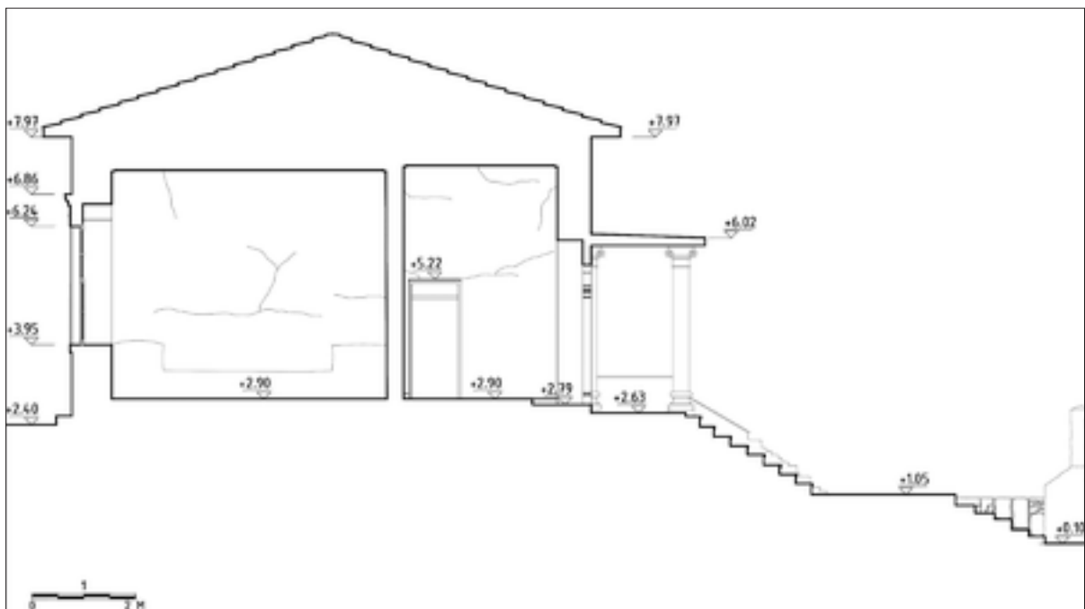
Şekil 9: 2-2 Kesiti.
