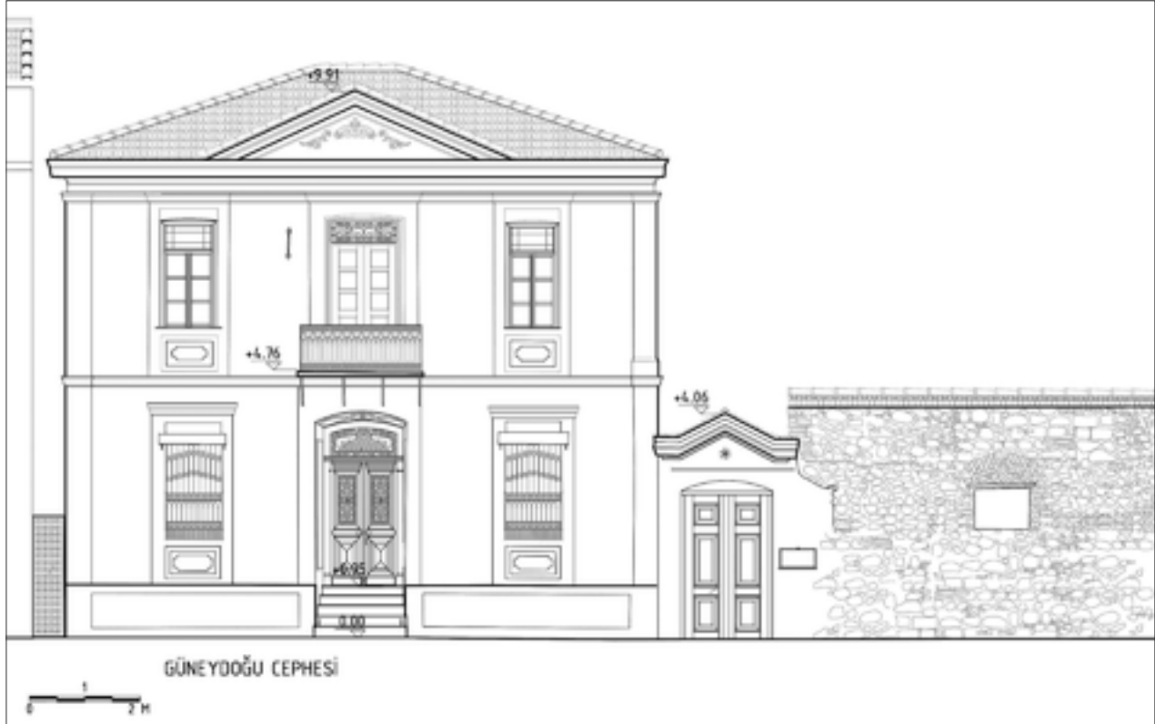
Şekil 22: Restorasyon ön cephe silüeti.
