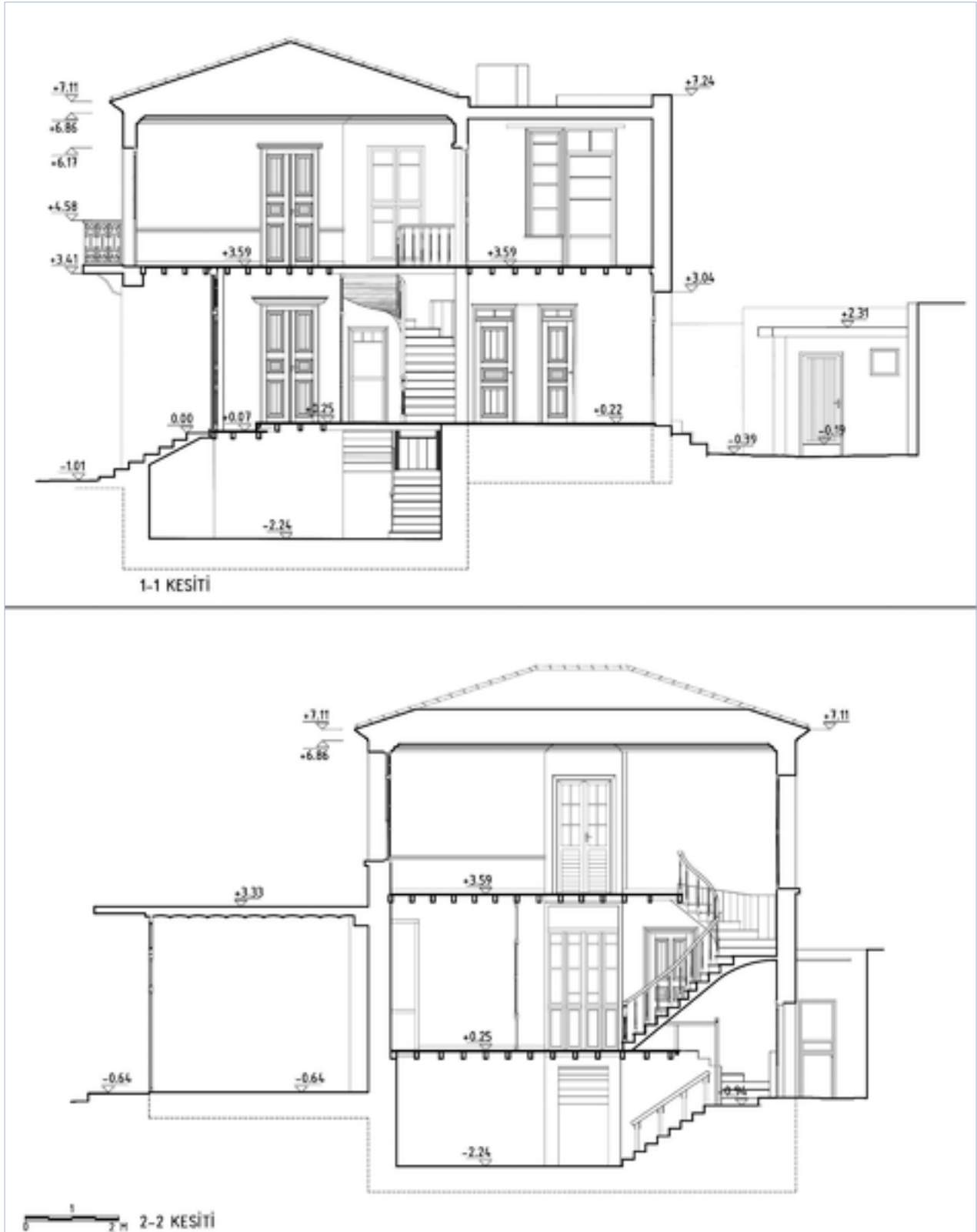
Şekil 20: Restorasyon kesitler.
