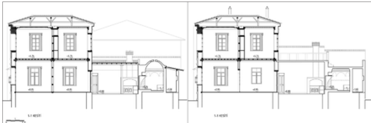
Şekil 16: I. dönem (solda) ve II. dönem (sağda) 1-1 Kesiti.
