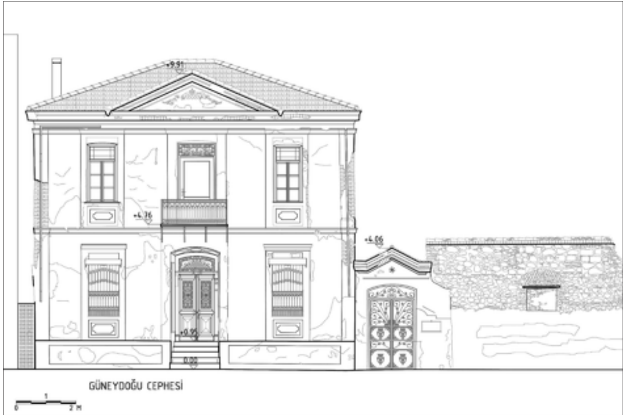
Şekil 9: Rölöve ön cephe silüeti.
