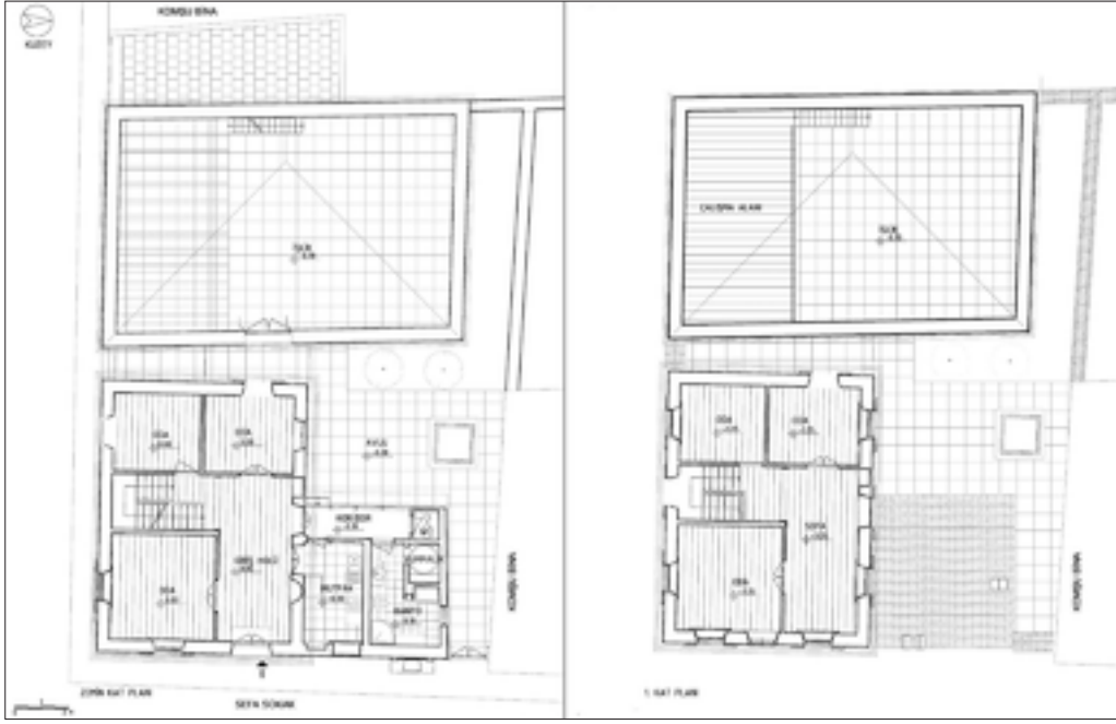
Şekil 13: Restorasyon kat planları.
