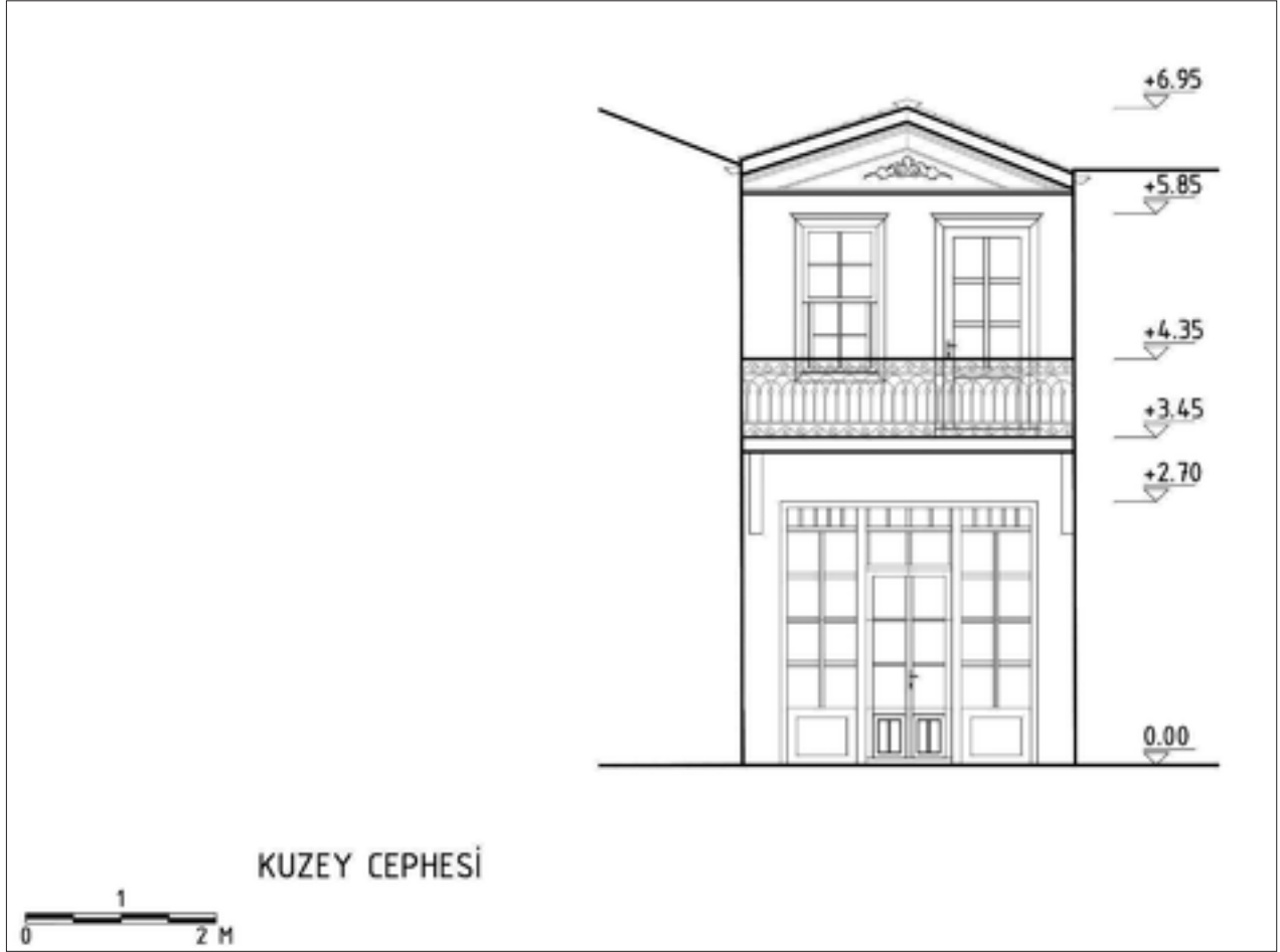
Şekil 9: Giriş cephe restitüsyon önerisi.
