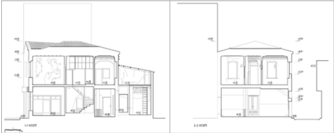
Şekil 6: Rölöve kesitler.
