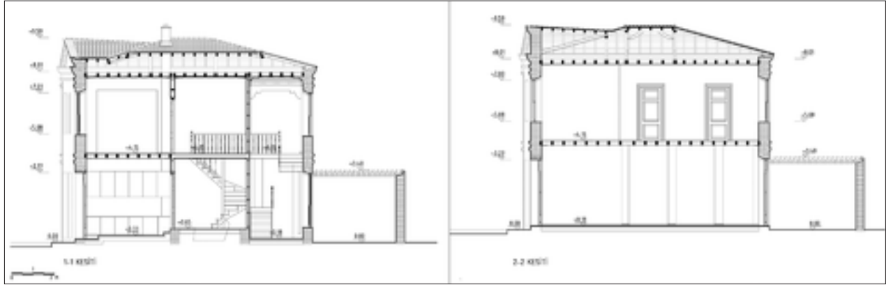
Şekil 13: Restorasyon kesitler.
