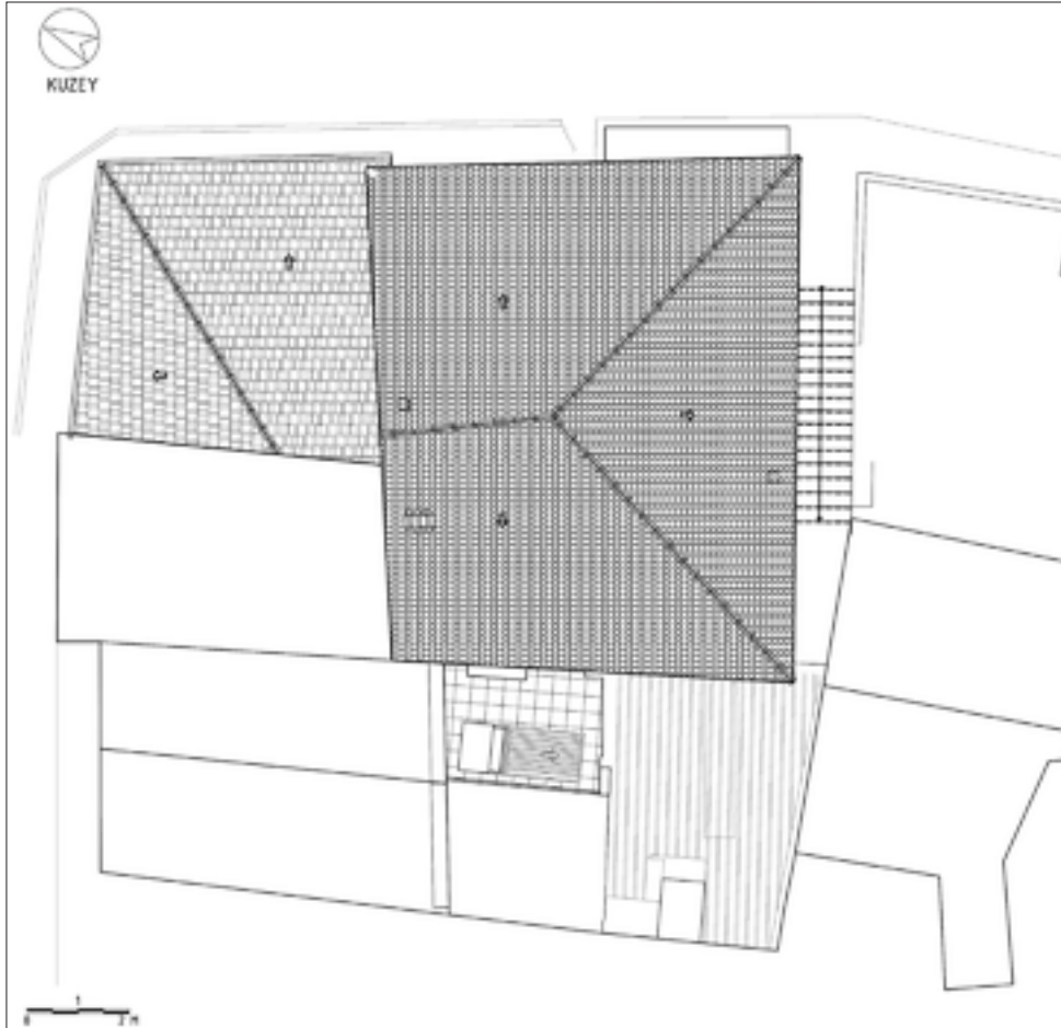
Şekil 11: Çatı rölöve planı.
