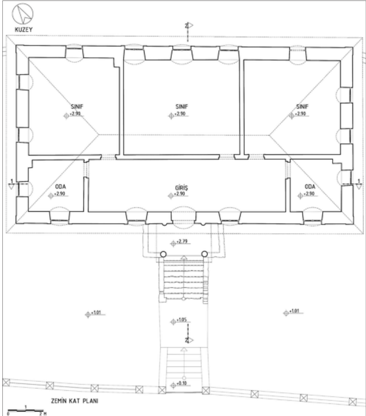
Şekil 7: Zemin kat (+2.90 kotlu) planı.
