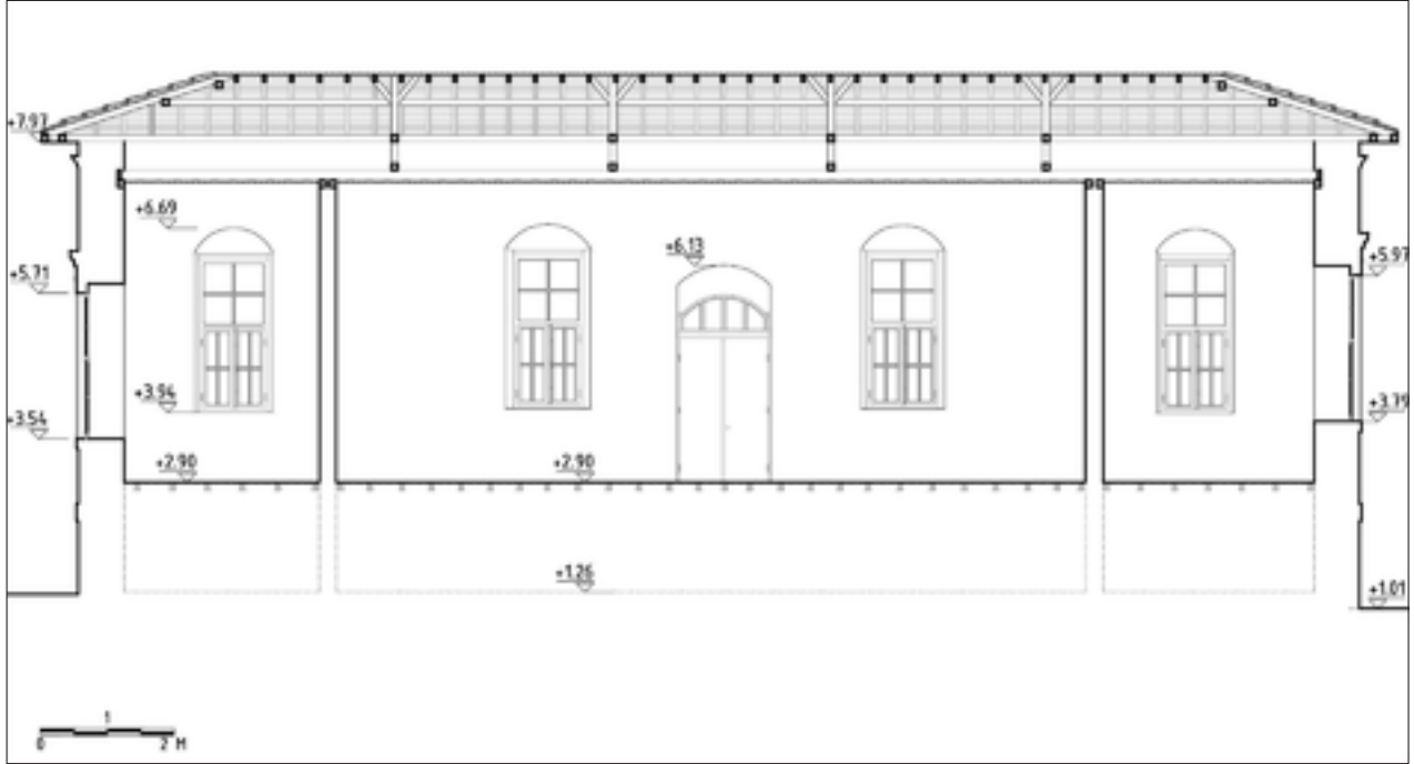
Şekil 15: Restitüsyon 2-2 kesiti.
