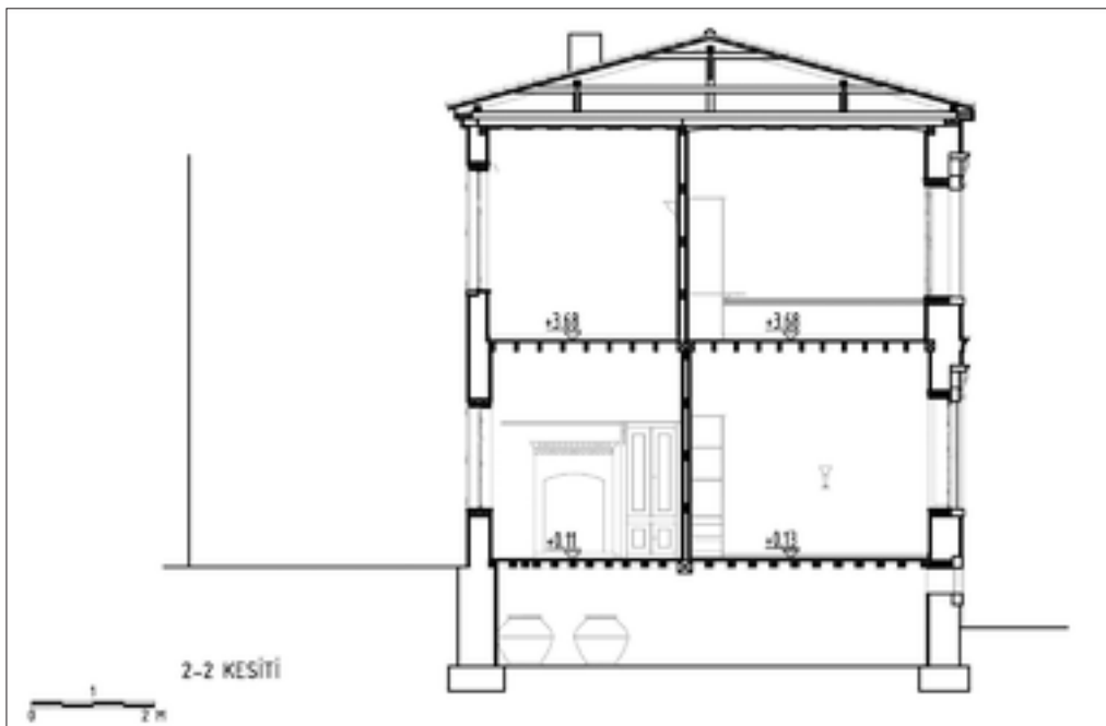
Şekil 16: 2-2 kesiti I. dönem restitüsyon önerisi.
