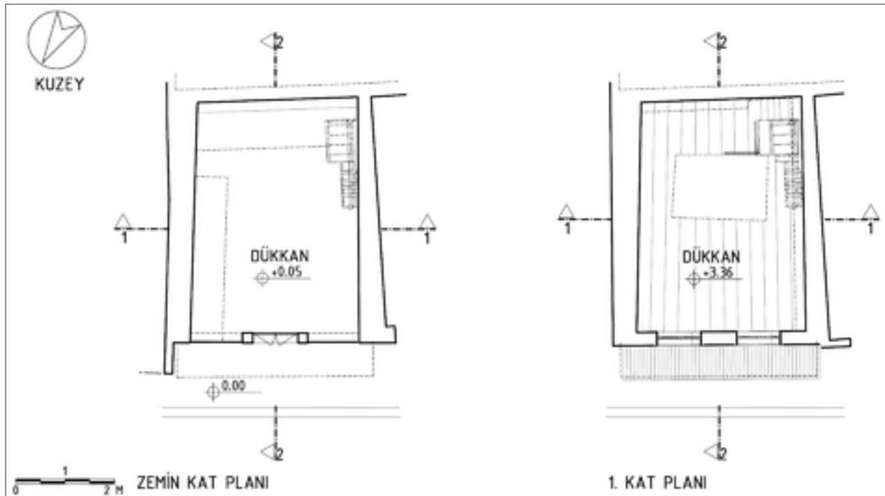
Şekil 4: Rölöve kat planları.
