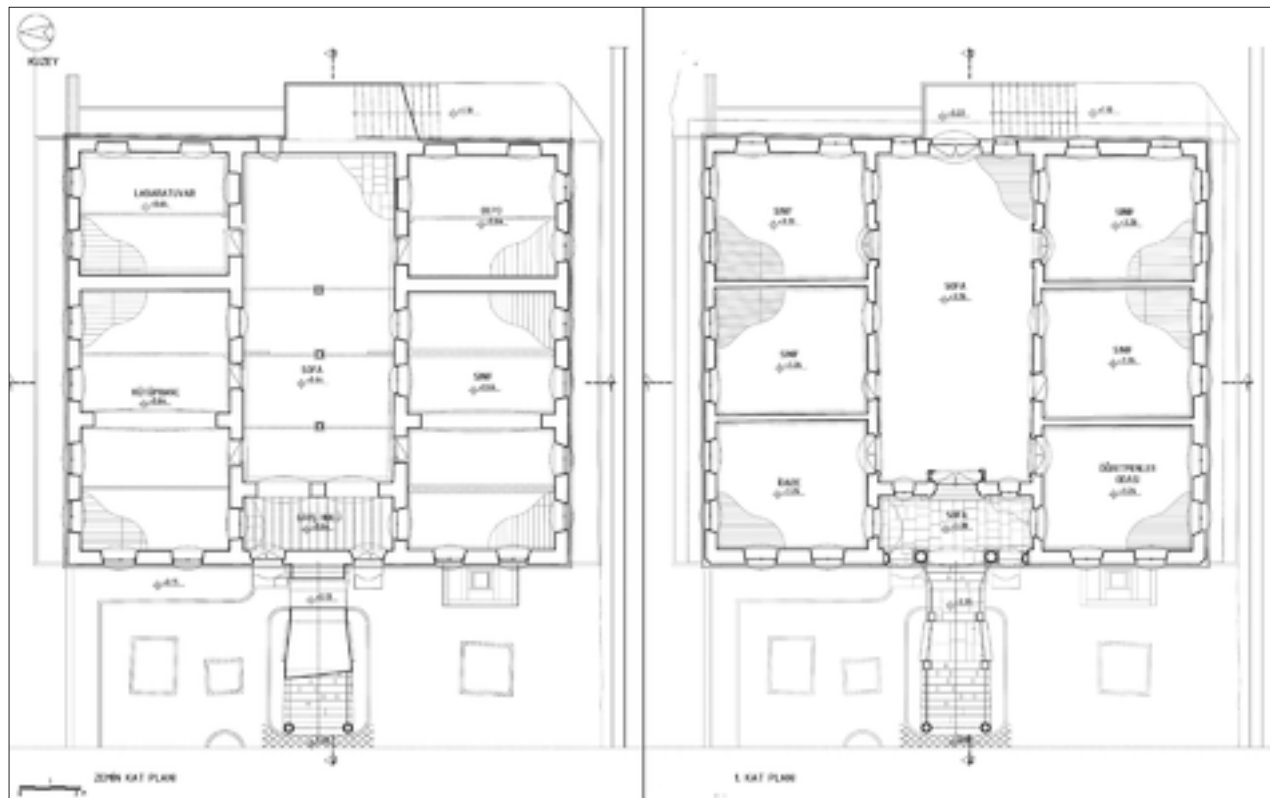
Şekil 17: Zemin ve birinci kat plan restorasyonu.
