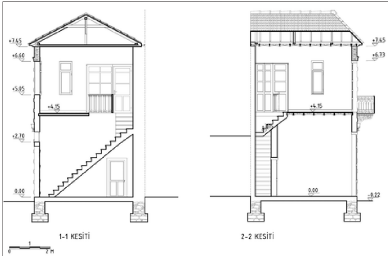
Şekil 7: Restitüsyon kesitler.
