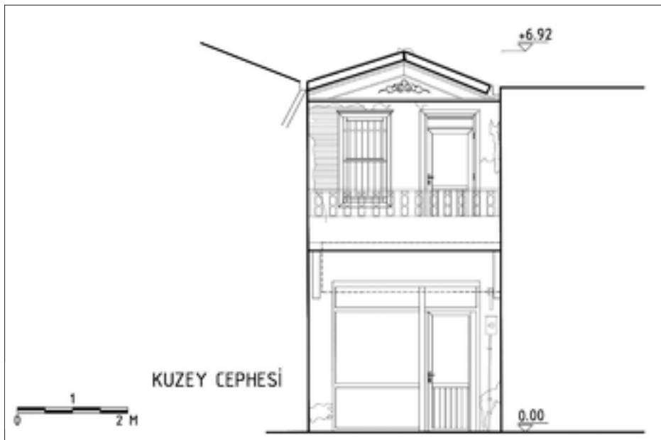
Şekil 7: Mevcut durum (rölöve) giriş cephesi.
