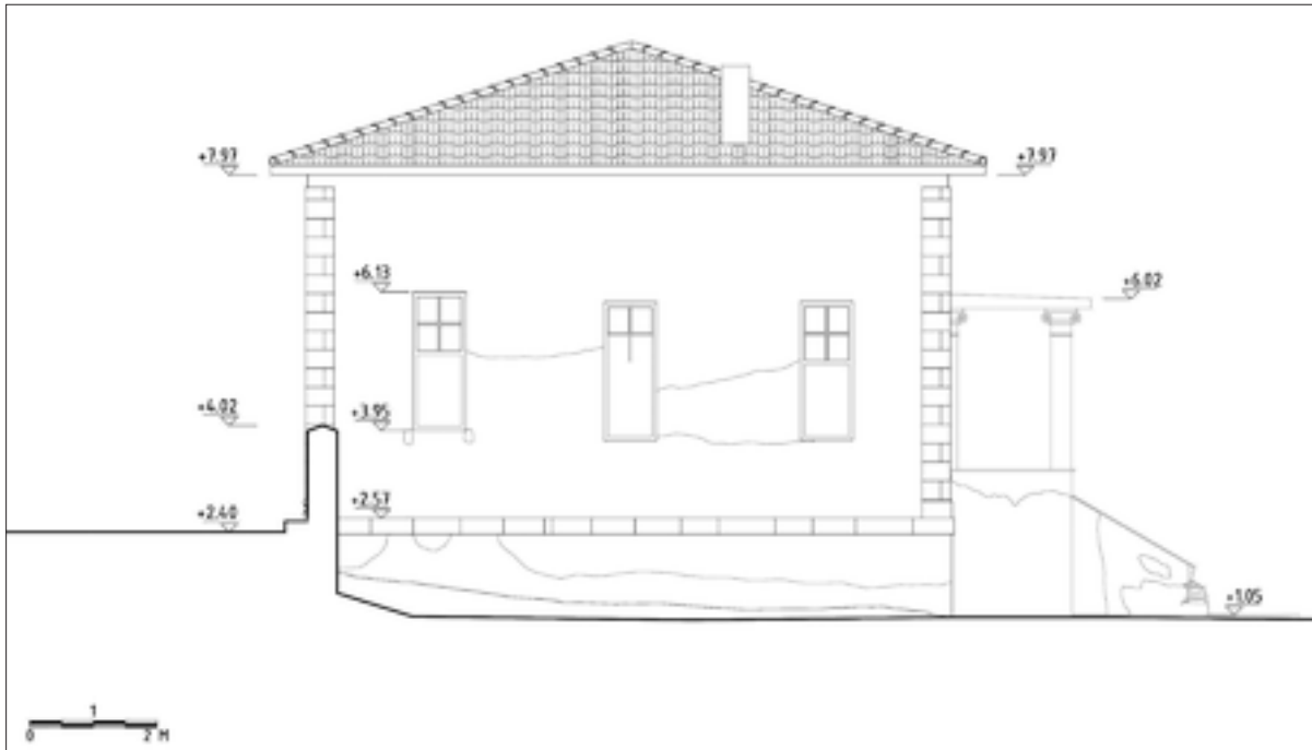
Şekil 12: Yan (doğu) cephe.
