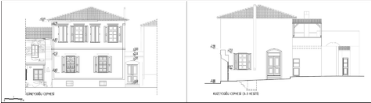
Şekil 16: Restorasyon cepheler.
