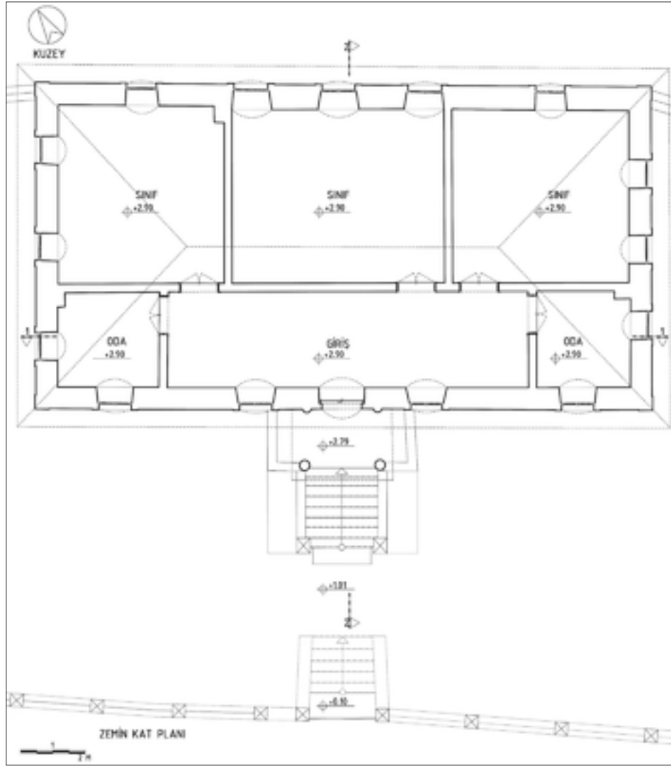
Şekil 13: Zemin kat (+2.90 kotlu) restitüsyon planı.
