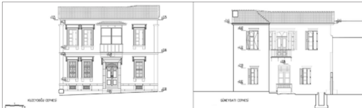
Şekil 12: Ön ve arka cepheler I. dönem restitüsyon önerisi.
