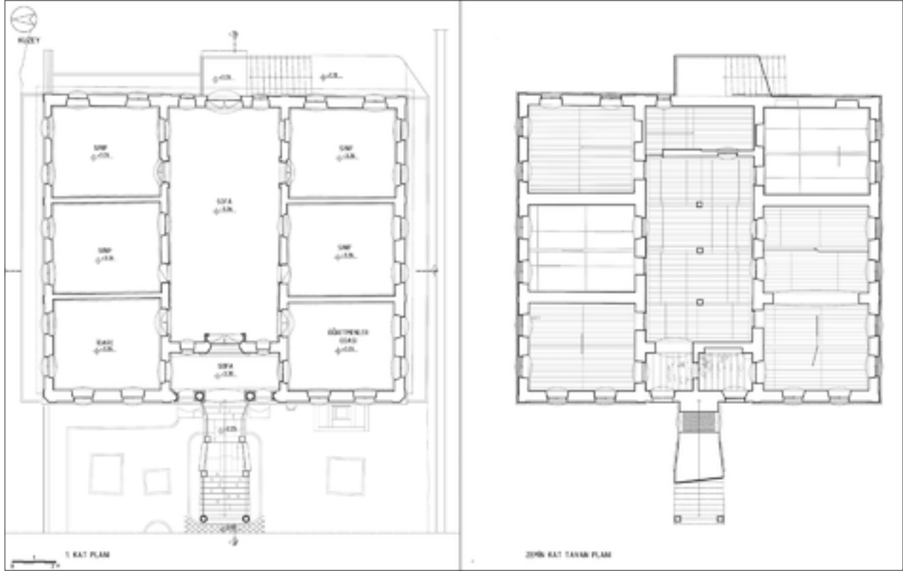
Şekil 5: Birinci kat plan ve tavan rölövesi.
