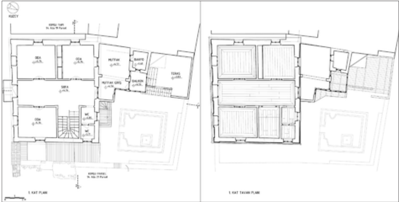
  ekil 8: R  l  ve birinci kat ve tavan planı.
