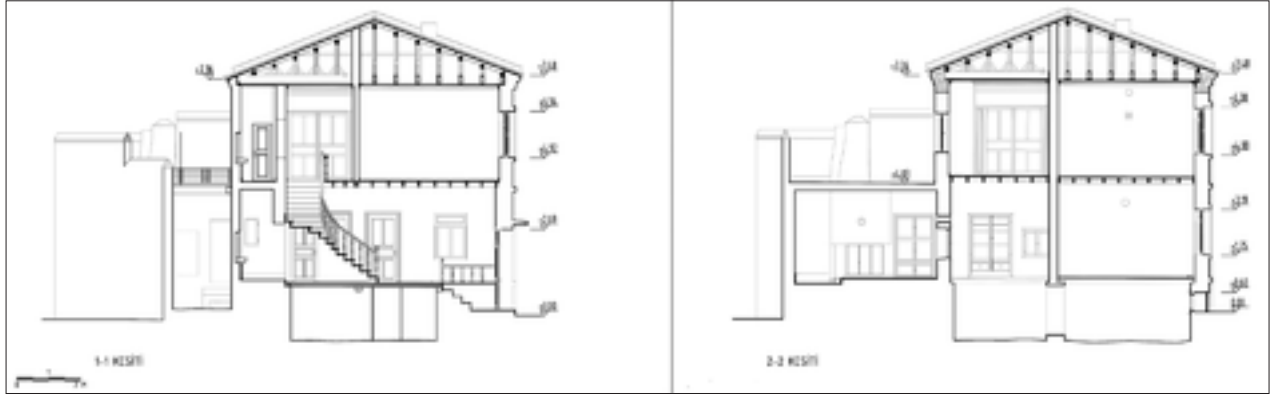
Şekil 7: Restitüsyon kesitler.
