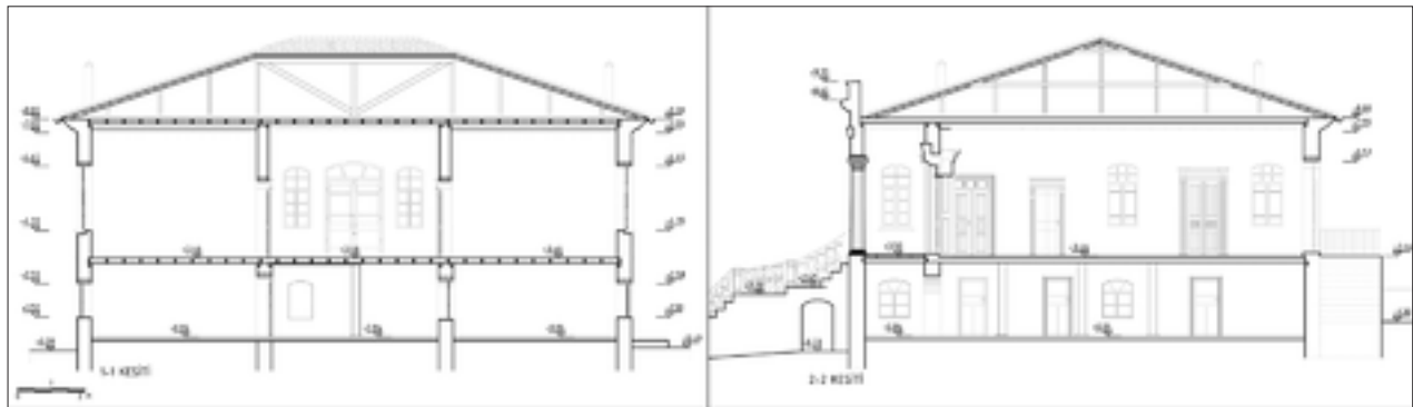
Şekil 13: 1-1 ve 2-2 kesit restitüsyon önerisi.
