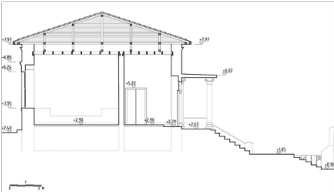
Şekil 14: Restitüsyon 1-1 kesiti.
