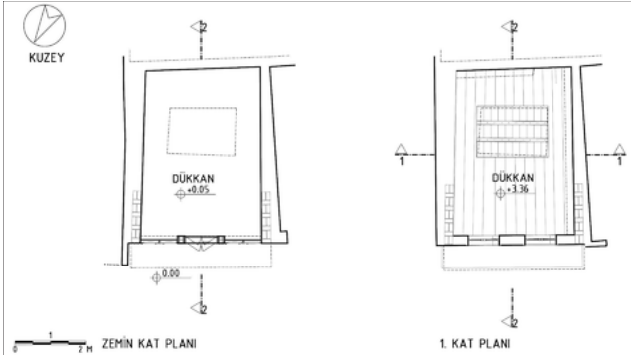
Şekil 10: Restorasyon kat planları.
