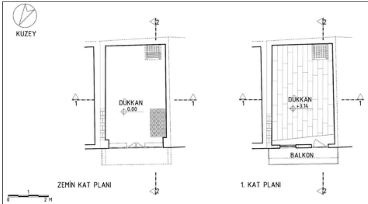
Şekil 11: Restorasyon kat planları.
