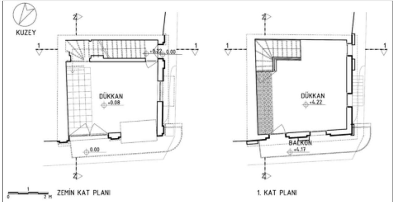
Şekil 3: Zemin ve birinci kat rölöve planları.
