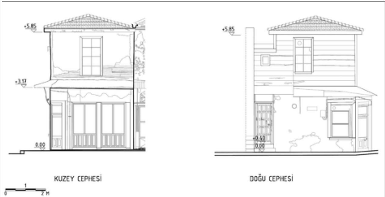
Şekil 6: Rölöve kuzey cephesi ve doğu cephesi.
