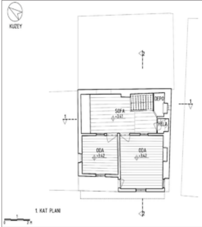
Şekil 9: 1. Kat planı.
