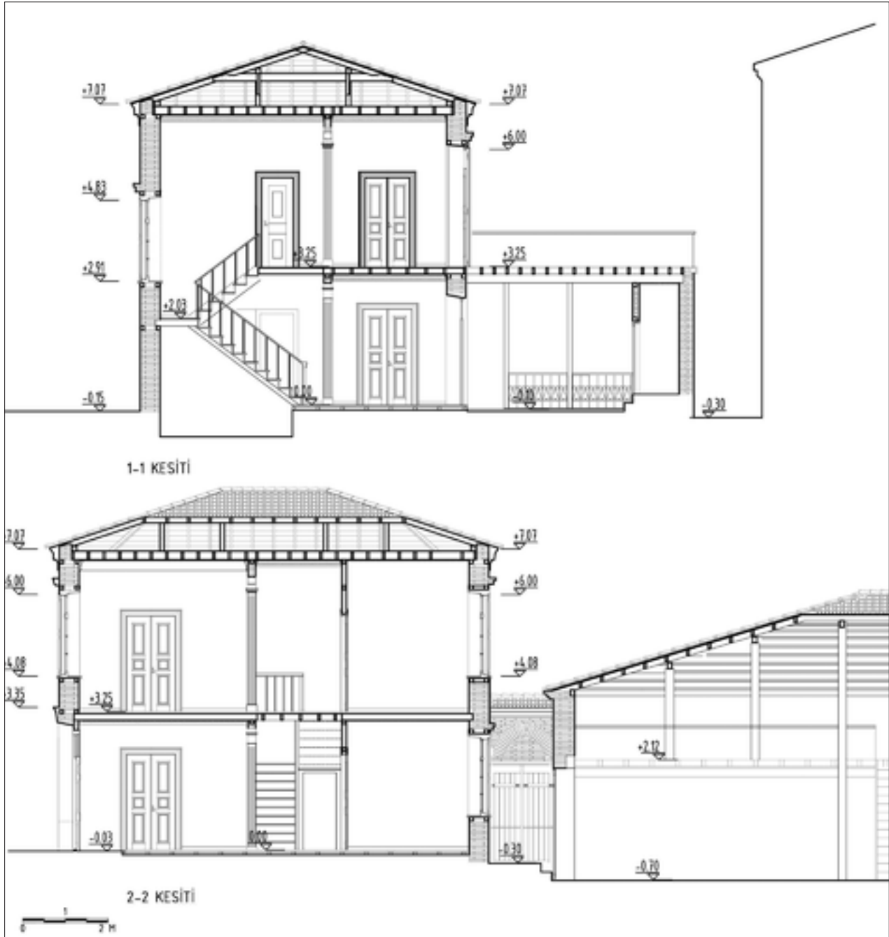
Şekil 11: Restitüsyon enine ve boyuna kesit.
