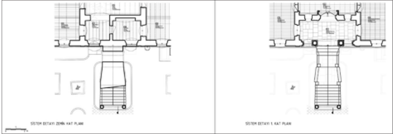
Şekil 10: Zemin kat ve birinci kat sistem detayı plan rölövesi.
