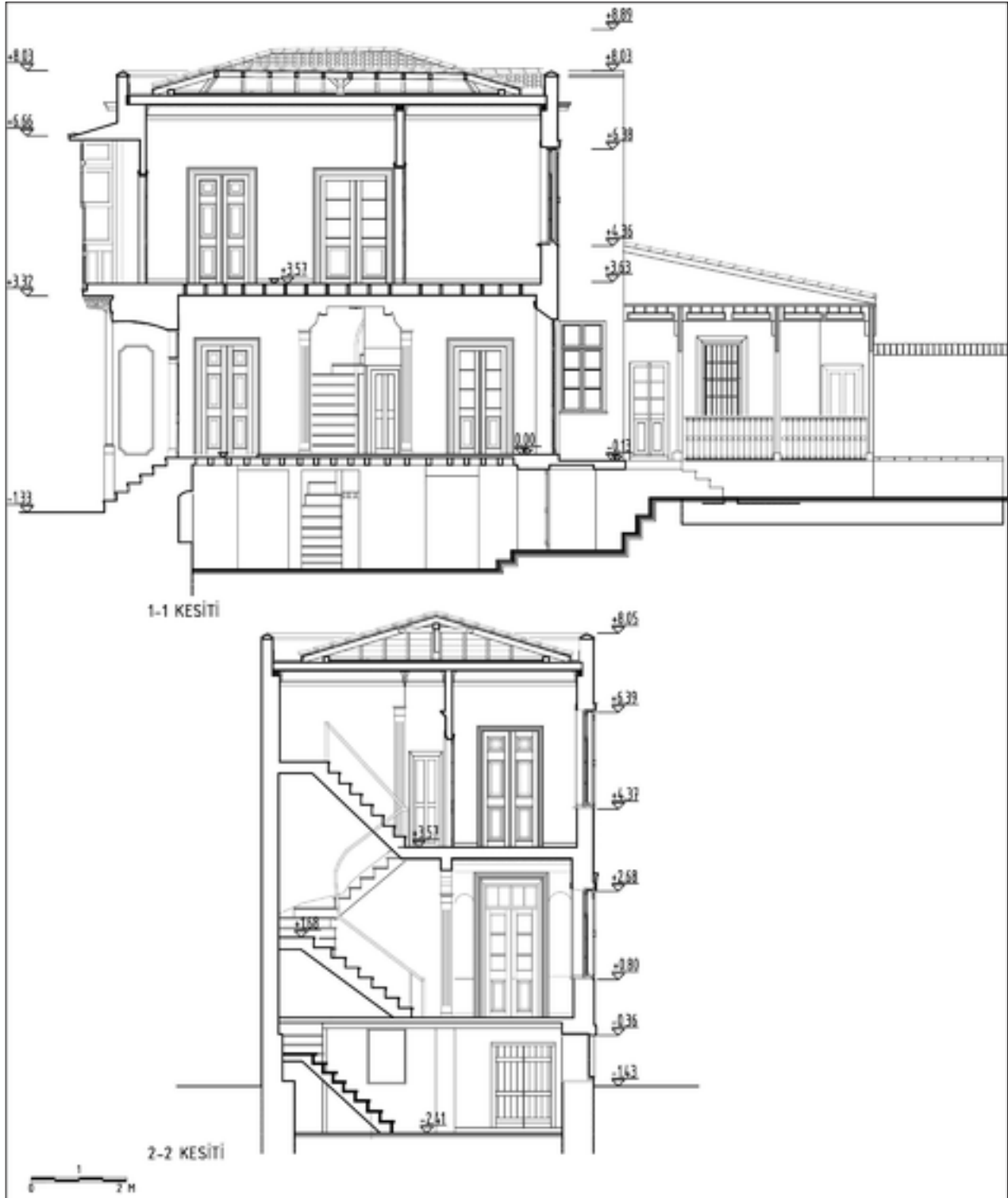
řekil 13: Restorasyon enine ve boyuna kesit.
