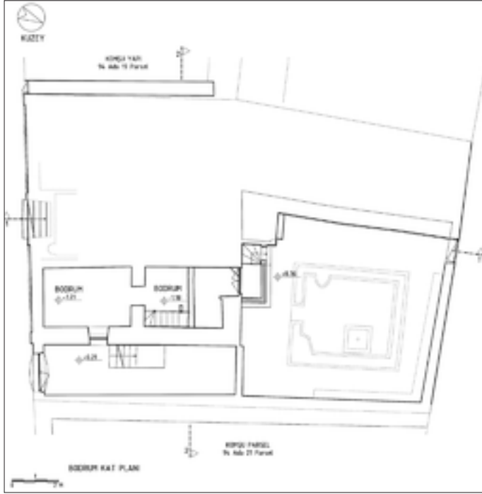
Şekil 3a: Bodrum kat planı.
