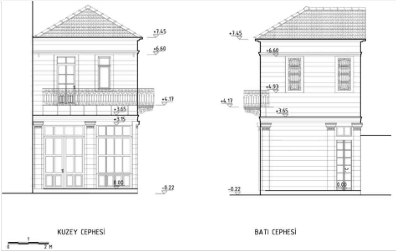
Şekil 11: Kuzey (Cumhuriyet Caddesi) ve batı cephesi restorasyon cephesi.
