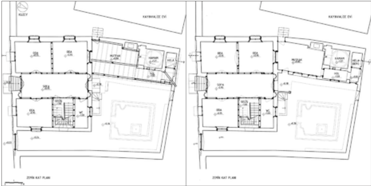
řekil 13: I. d  nem (solda) ve II. d  nem (sa  da) restit  syon zemin kat planı.
