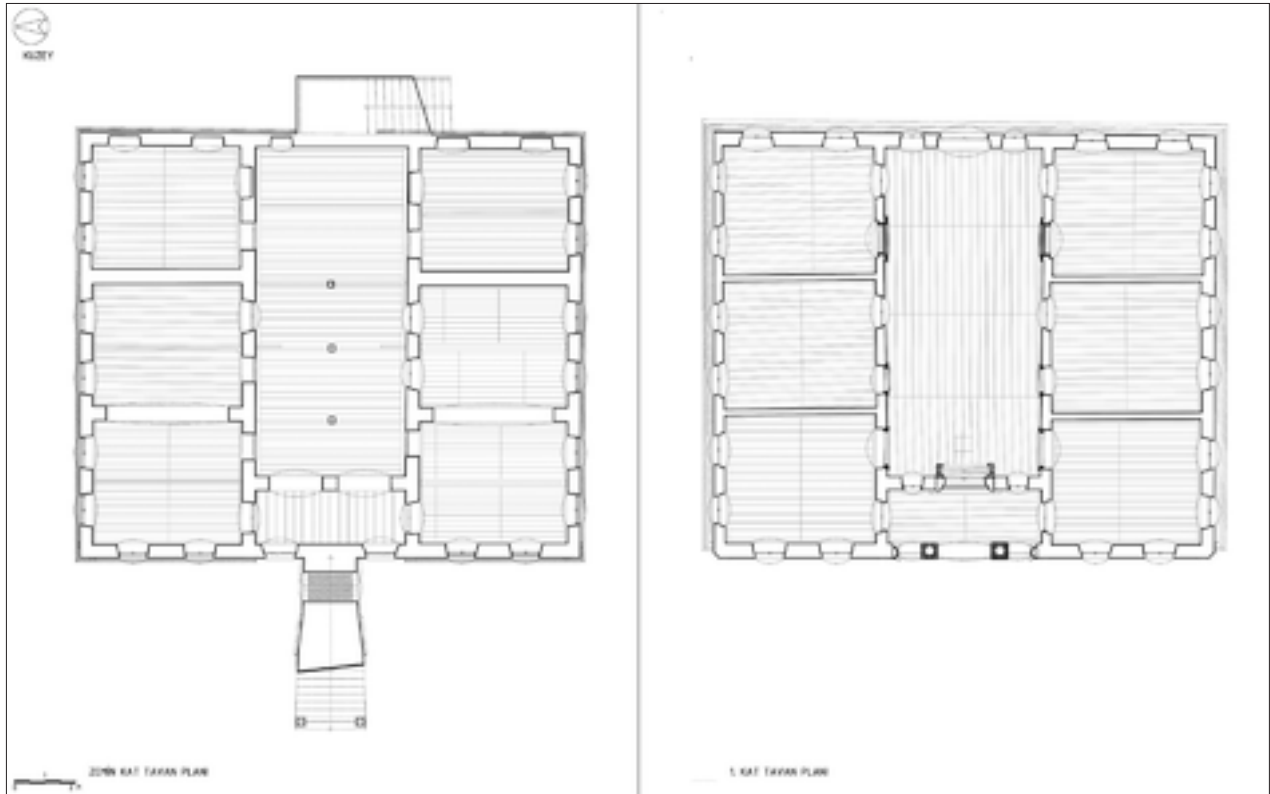
Şekil 12: Zemin ve birinci kat tavan planları restitüsyon önerisi.
