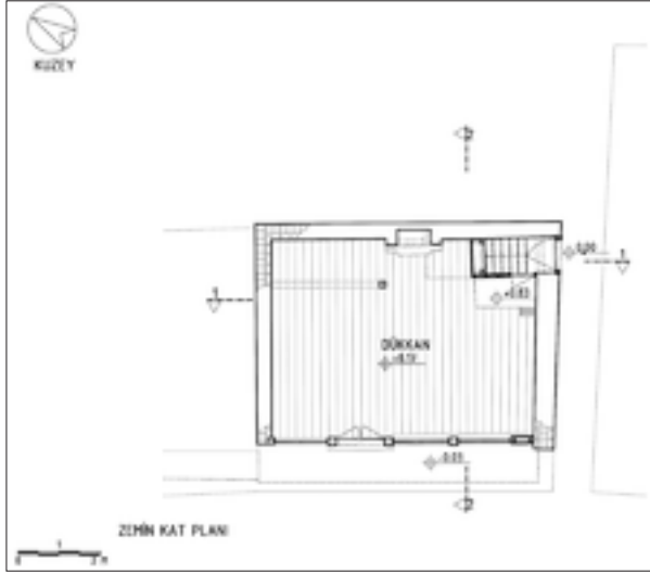
Şekil 20: Zemin kat planı.
