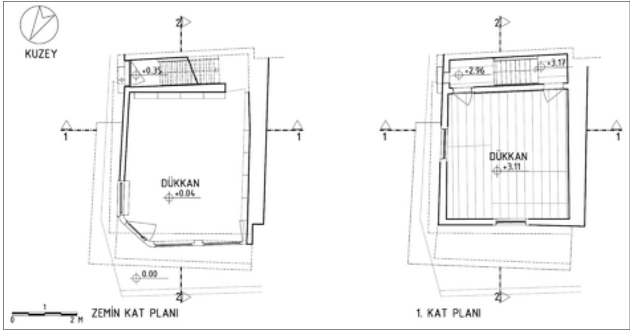
Şekil 5: Rölöve kat planları.
