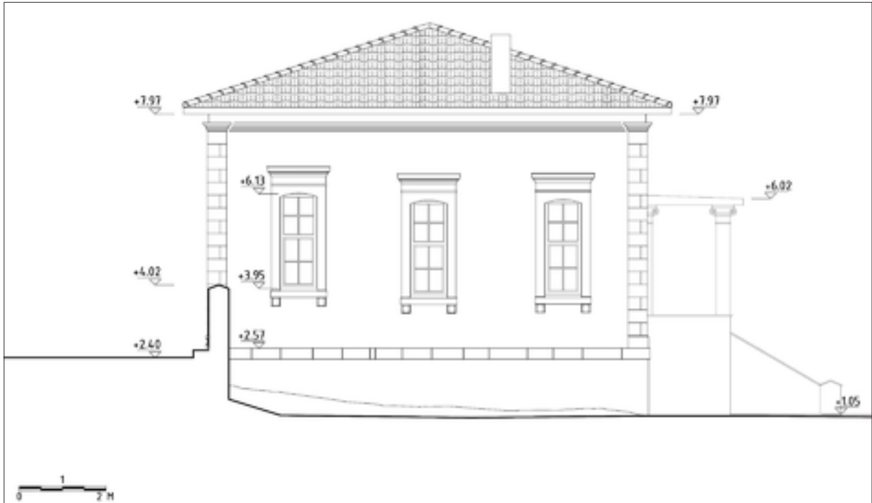
Şekil 18: Restitüsyon projesi yan (doğu) cephe.
