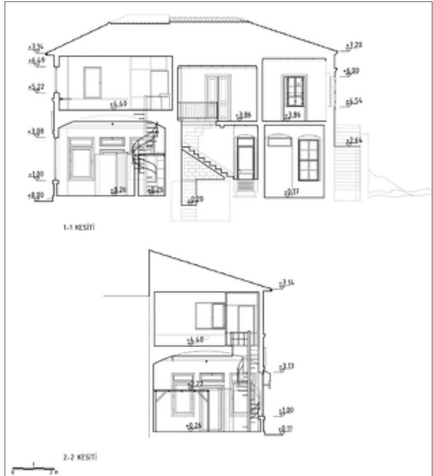
Şekil 12: Kesit rölöveleri.
