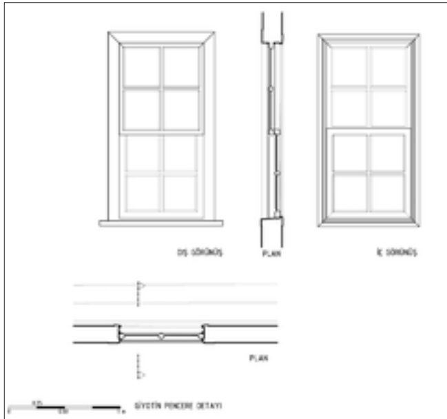
Şekil 18: Batı cephe giyotin pencere detayı çizimi.
