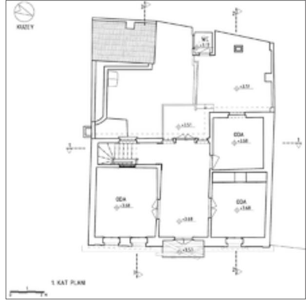
Şekil 4: Birinci kat plan rolövesi.
