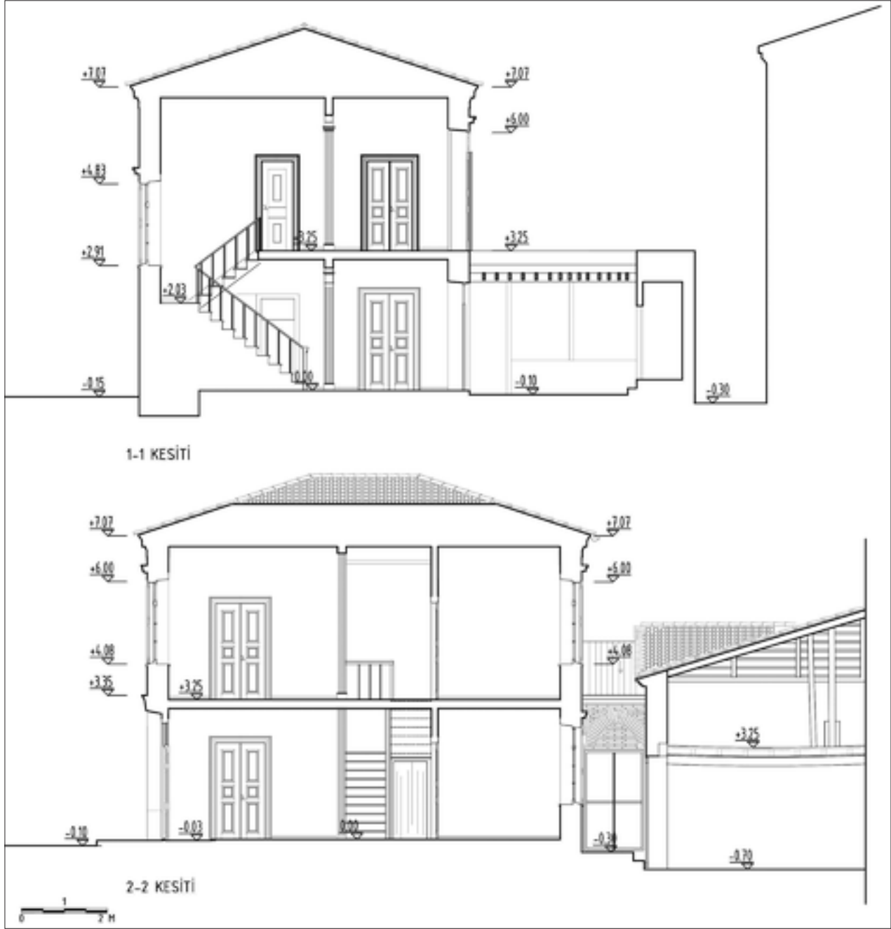
Şekil 8: Rölöve enine ve boyuna kesit.
