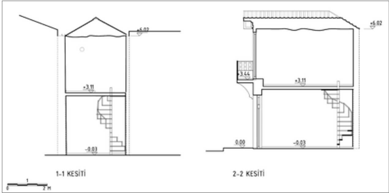
Şekil 6: Rölöve kesitler.
