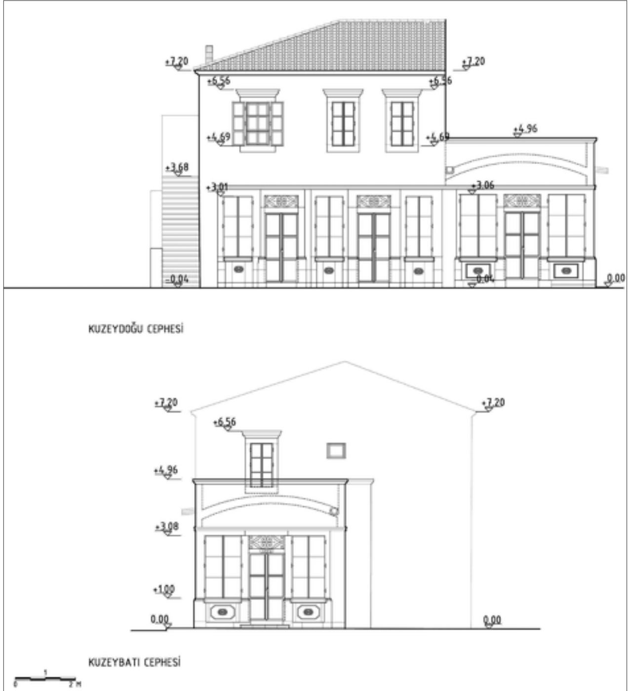
Şekil 18: Cephe restitüsyonu.
