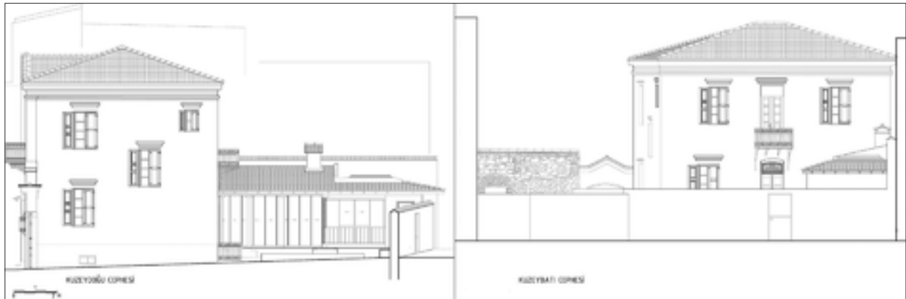
Şekil 23: Restorasyon sağ yan ve arka cephe.
