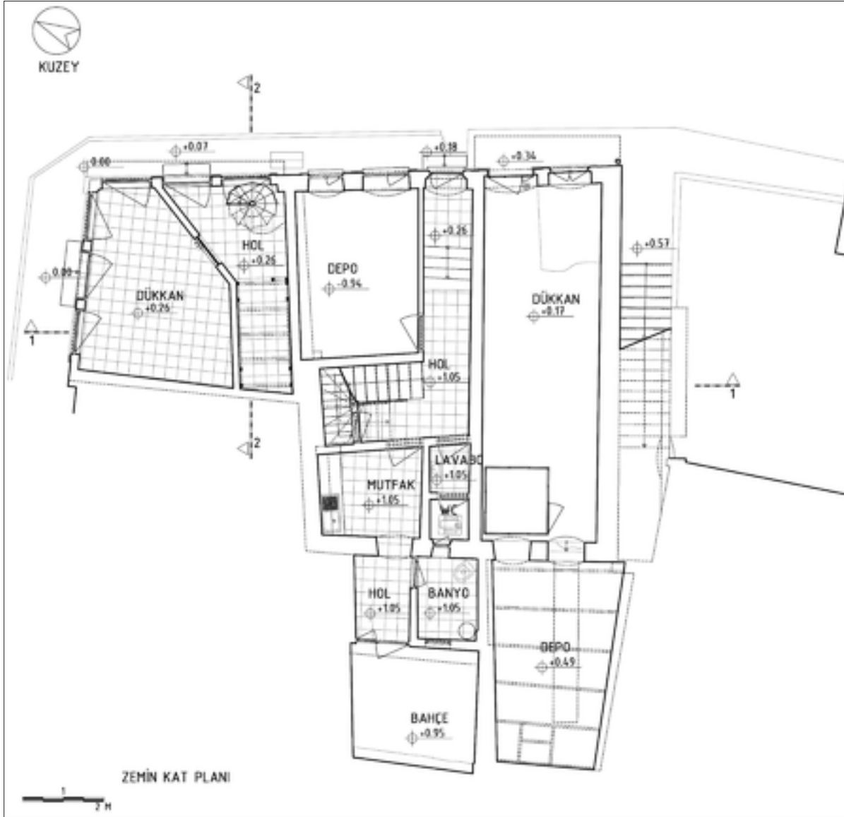
Şekil 9: Zemin kat rolöve planı.
