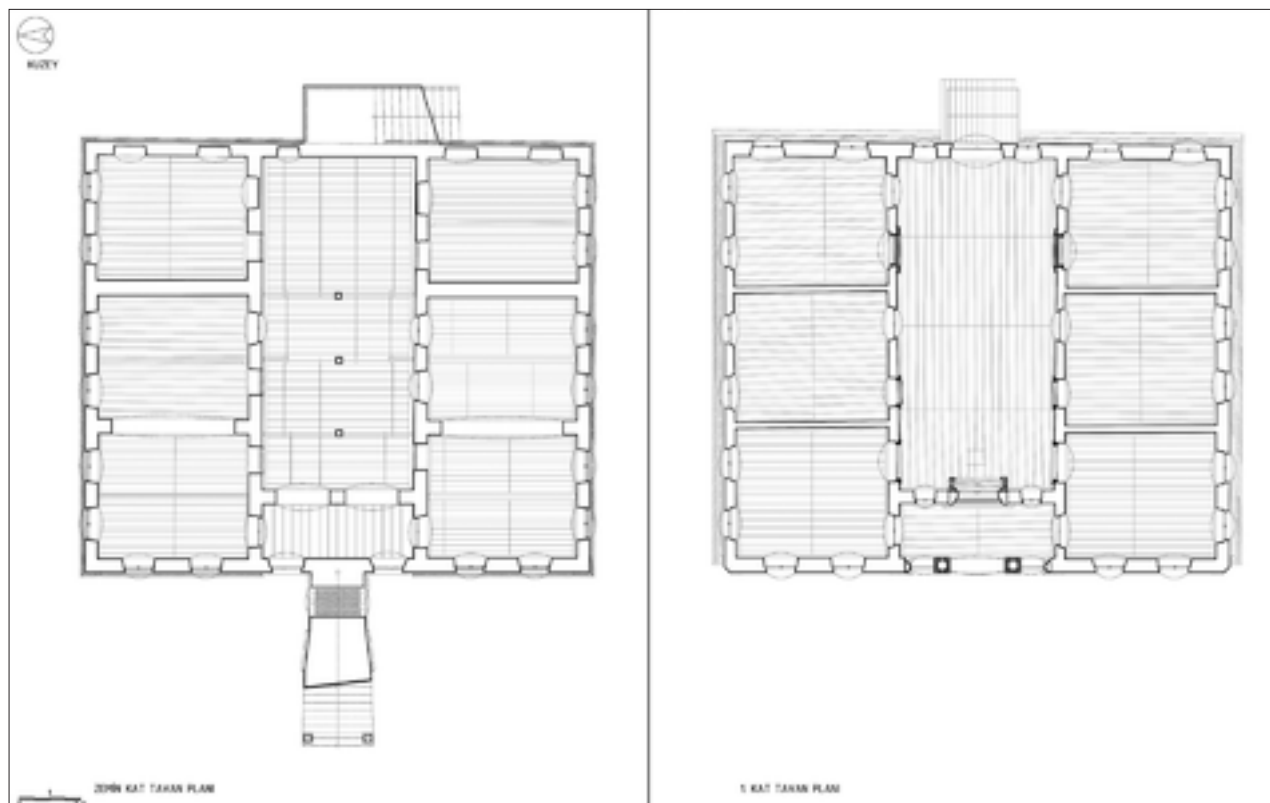
Şekil 18: Zemin ve birinci kat tavan planları restorasyonu.
