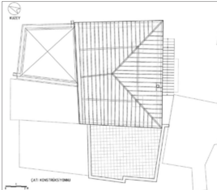
Şekil 16: Çatı konstrüksiyonu restitüsyon planı.
