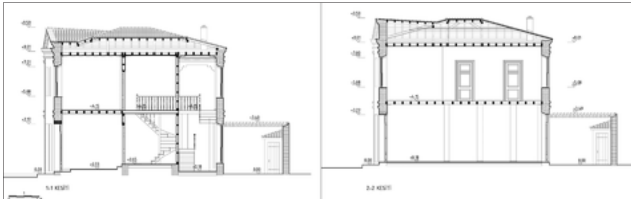
Şekil 9: Restitüsyon kesitler.
