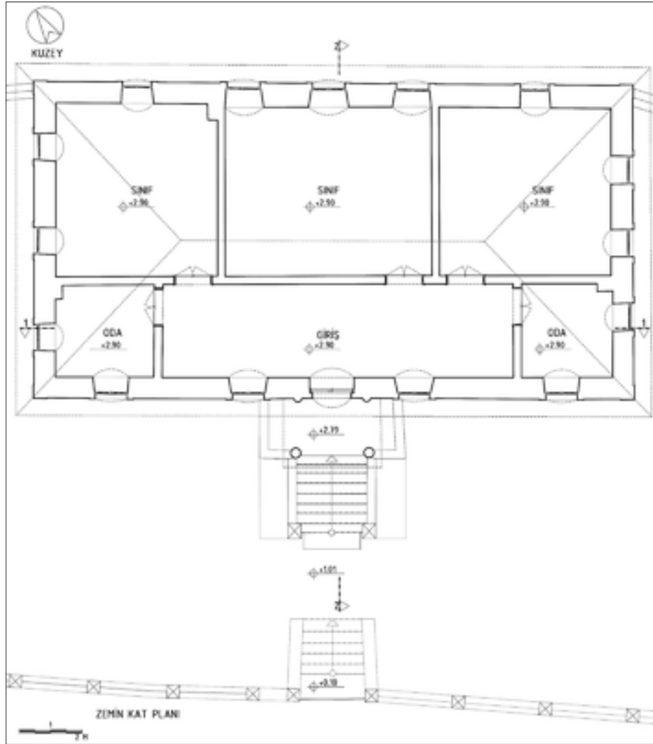
Şekil 19: Restorasyon önerisi zemin kat (+2.90 kotlu) planı.
