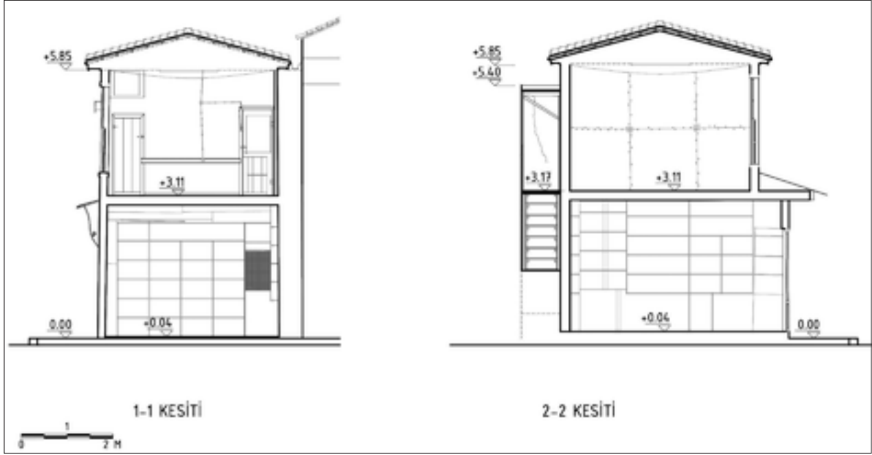
Şekil 7: Rölöve enine ve boyuna kesit.
