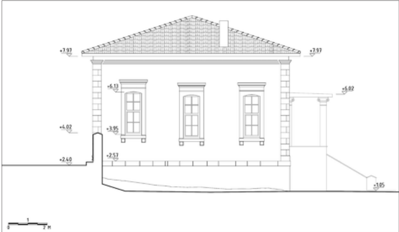
Şekil 24: Restorasyon önerisi yan (doğu) cephe.
