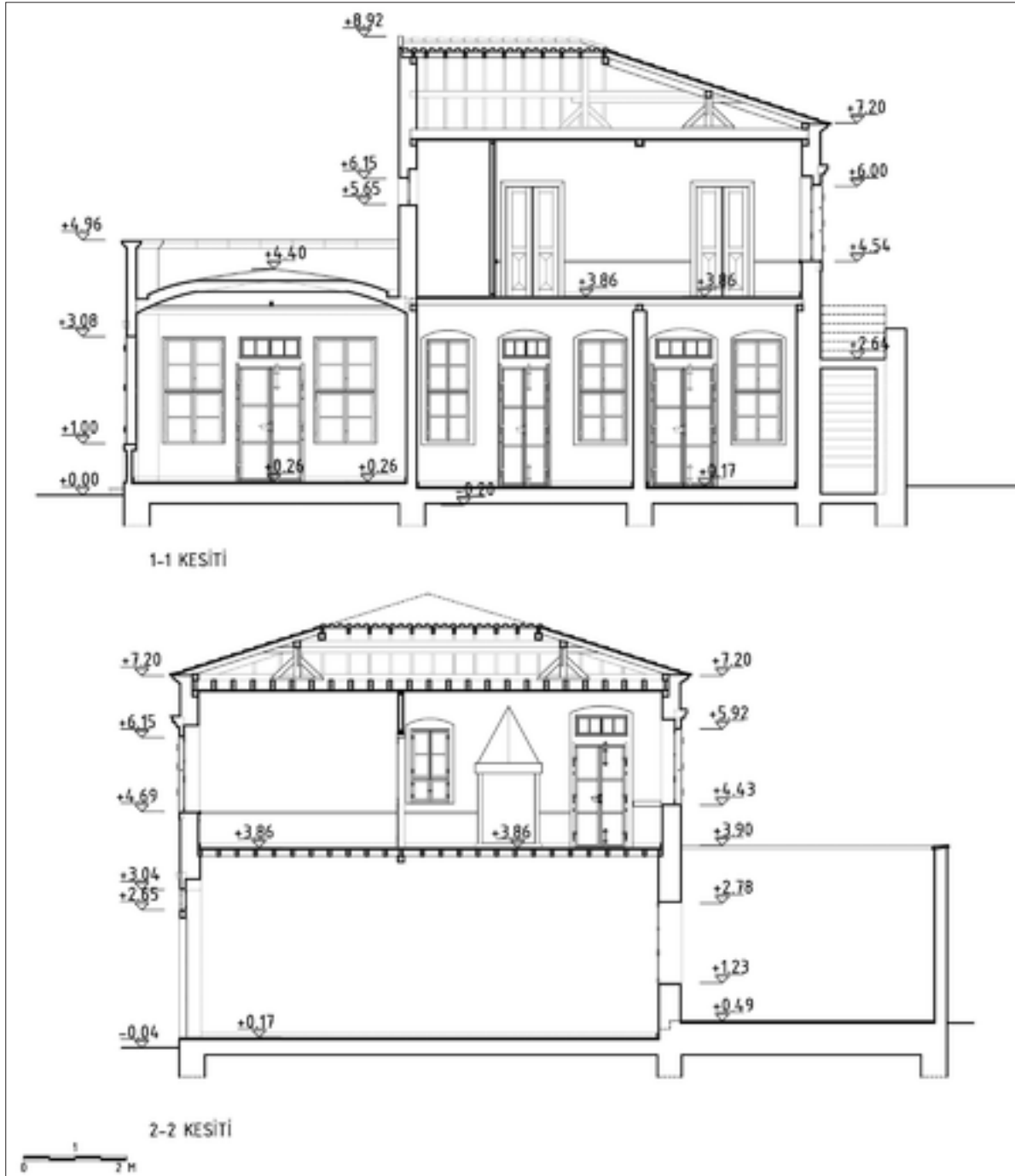
Şekil 17: Kesit restitüsyonu.
