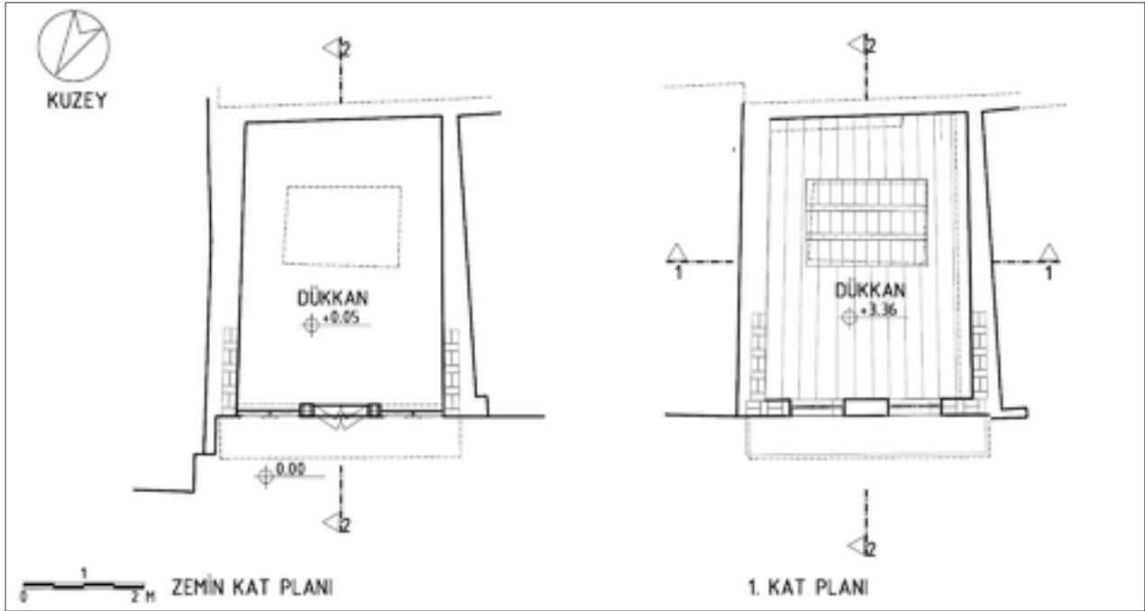
Şekil 7: Restitüsyon kat planları.
