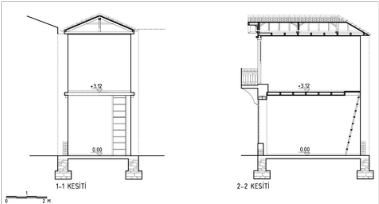
Şekil 10: Restitüsyon A-A ve B-B kesit önerisi.
