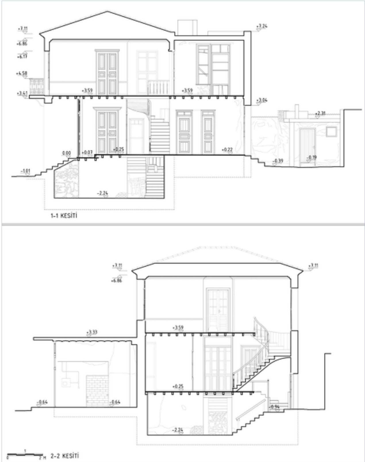
Şekil 11: Rölöve kesitler.
