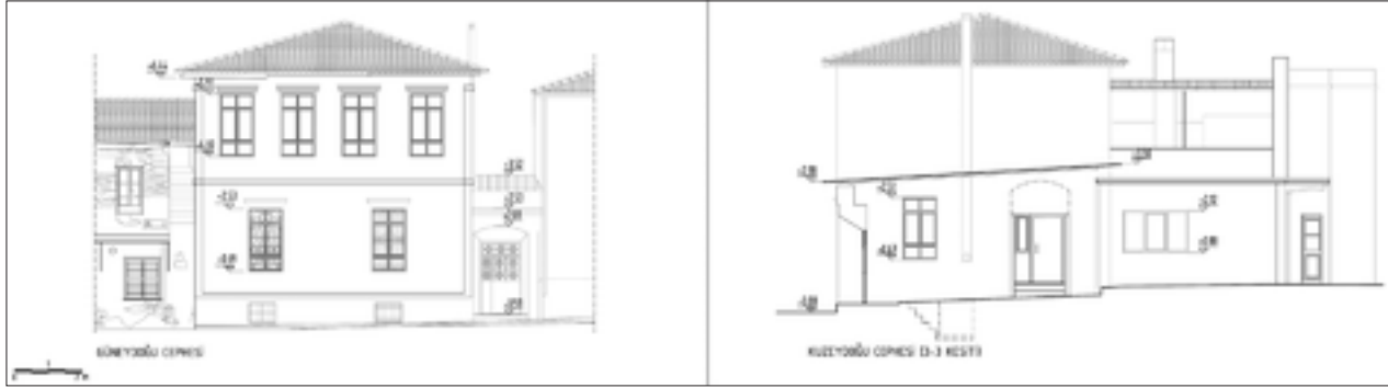
Şekil 9: Rölöve cepheler.
