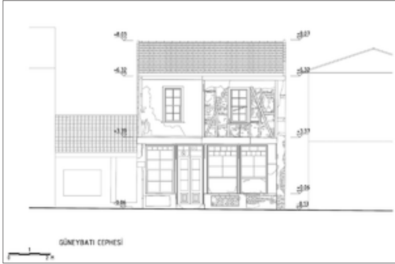
Şekil 12: Batı cephesi rölöve çizimi.
